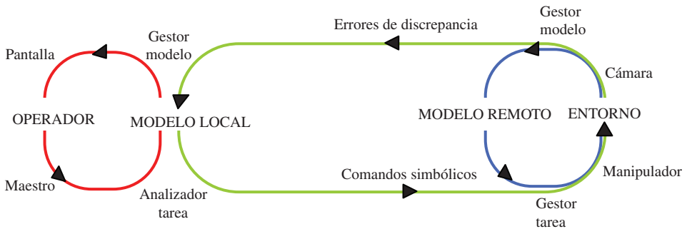
Figura 11.40. Lazos de control de la arquitectura de teleprogramación [HERNANDO-02].
