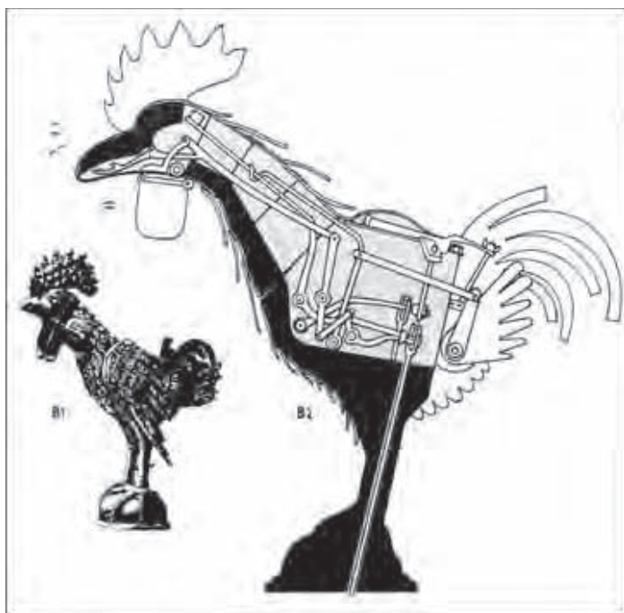
Figura 1.1. Gallo de Estrasburgo (1352).
