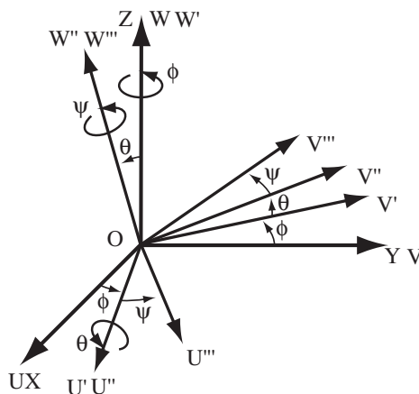
Figura 3.7. Ángulos de Euler WUW.
