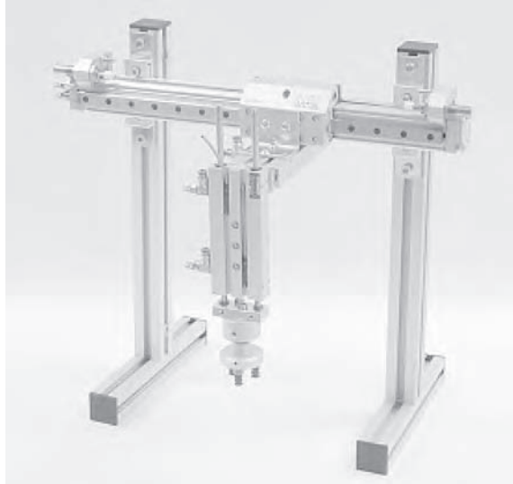
Figura 1.11. Manipulador secuencial neumático. (Cortesía FESTO).
