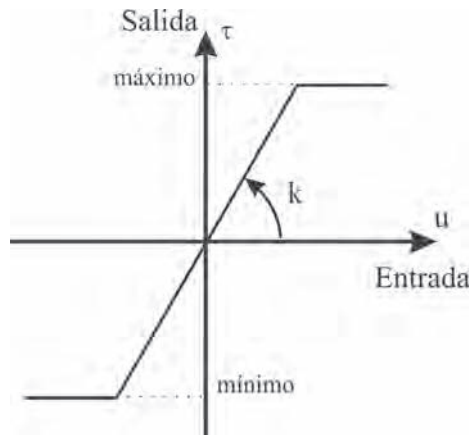
Figura 7.20. Relación entre entrada y salida de un amplificador con saturaciones.
