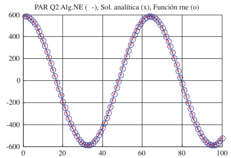
Figura 5.25. Trayectoria y Pares con primer gdl nulo y segundo en movimiento.
