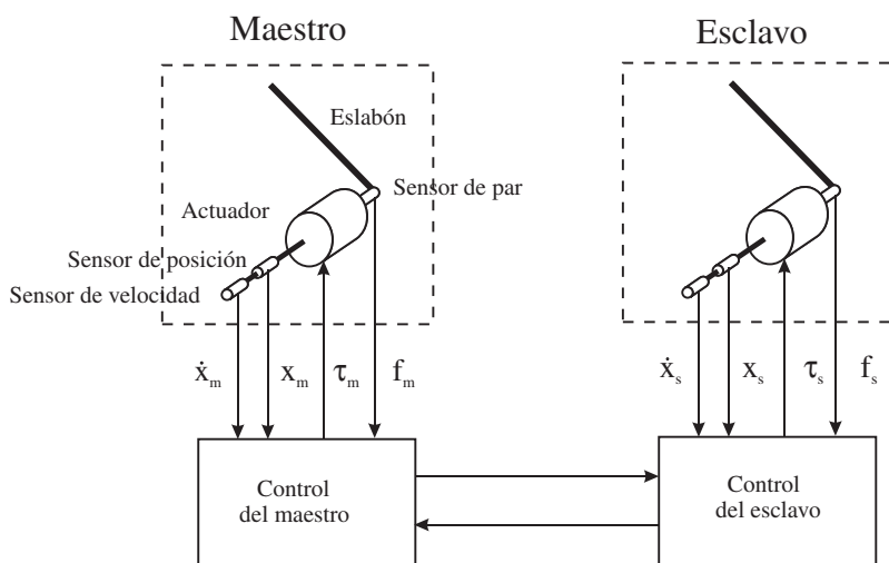
Figura 11.28. Esquema general de control bilateral.
