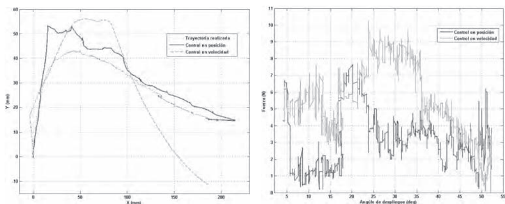
Figura 11.61. Comparación de los experimentos de plegado utilizando realimentación de fuerzas para guiar al operador. Trayectoria (izquierda) y fuerzas desarrolladas (derecha).
