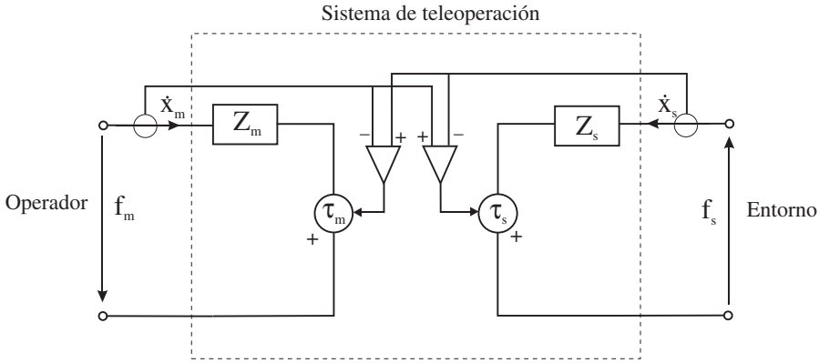
Figura 11.36. Control bilateral posición-posición mediante teoría del cuadripolo.
