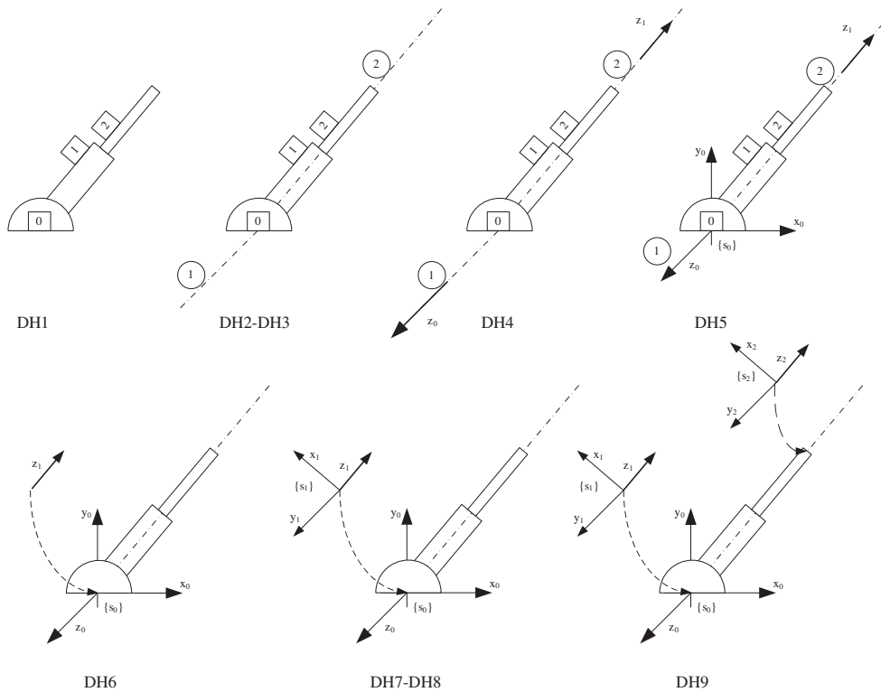
Figura 4.19. Secuencia del algoritmo de D-H para el robot del Ejercicio 4.1.
