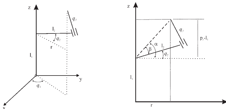
Figura 4.31. Solución mediante métodos geométricos del robot del Ejercicio 4.7.
