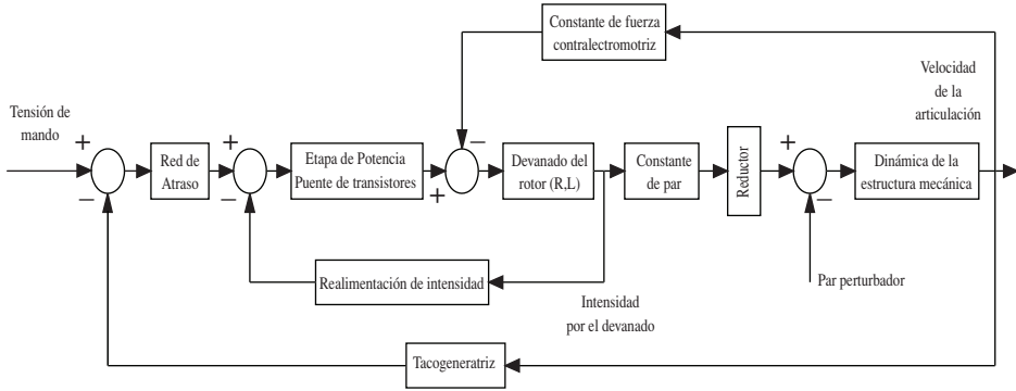
Figura 5.9. Esquema de bloques del modelo de un motor eléctrico de corriente continua.
