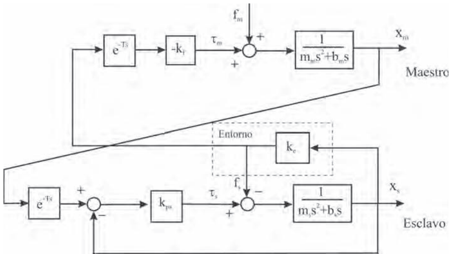
Figura 11.65. Diagrama de bloques del esquema de control bilateral fuerza-posición con retrasos en las comunicaciones.
