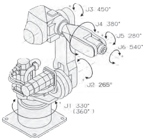
Figura 2.6. Grados de libertad del robot ARC Mate 120/S-12. (Cortesía de FANUC).
