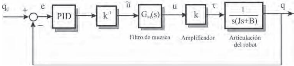
Figura 7.26. Control monoarticular con la inclusión de un filtro de muesca.
