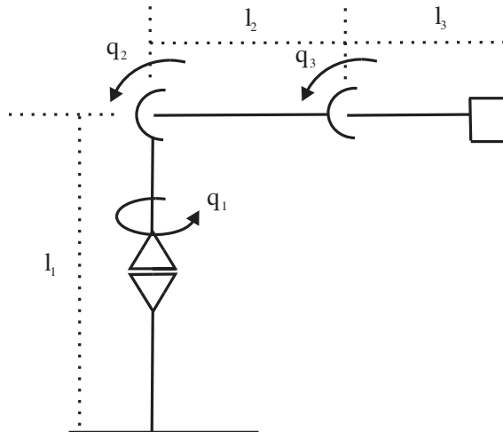
Figura 4.28. Modelo simplificado del robot de la Figura 4.9.
