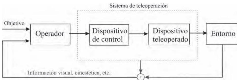
Figura 11.14. El operador como controlador del sistema de teleoperación.
