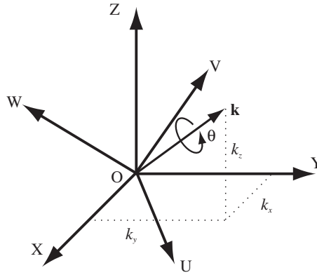
Figura 3.10. Representación de orientación por eje y ángulo de giro (par de rotación).
