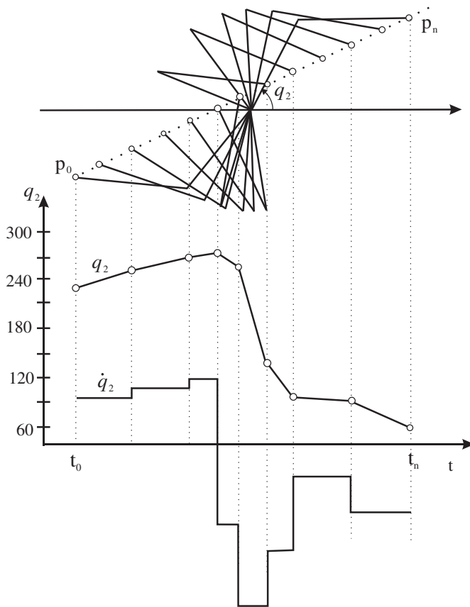
Figura 4.17. Ejemplo de punto singular para un robot tipo SCARA.
