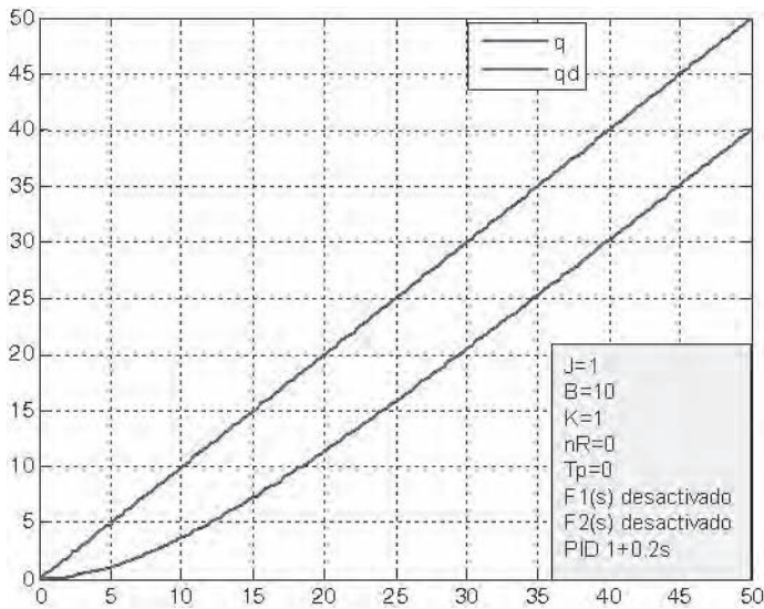
Figura 7.41. Trayectoria deseada q_d y real q ante entrada en rampa con control PD.
