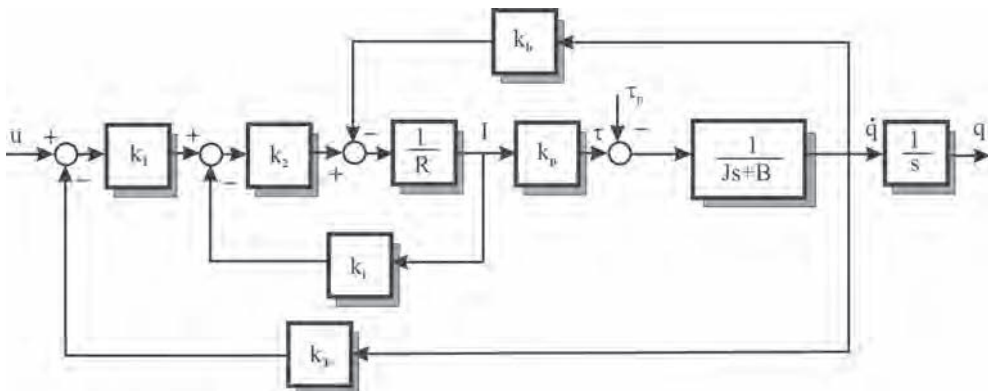
Figura 7.4. Diagrama de bloques de un accionamiento eléctrico.
