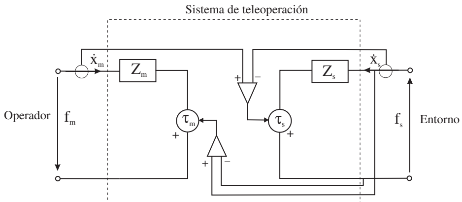
Figura 11.64. Representación del sistema de control bilateral fuerza-posición mediante la teoría del cuadripolo.
