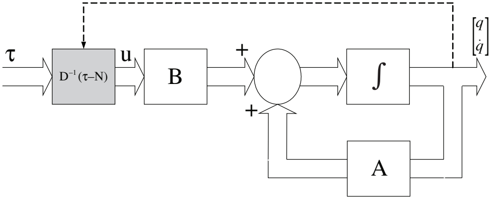
Figura 5.7. Diagrama de bloques de la dinámica de un robot en el espacio de estado.
