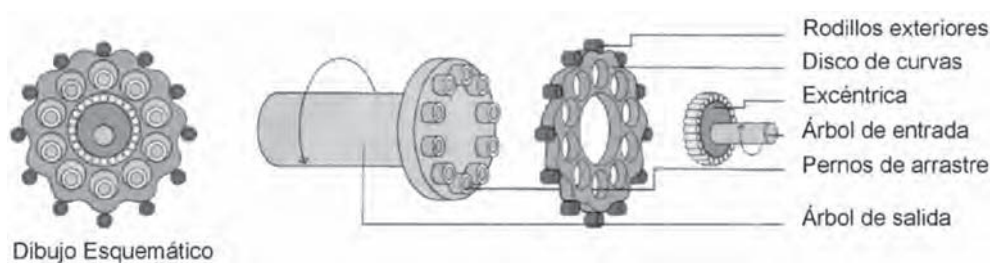
Figura 2.11. Reductor cíclico. (Cortesía de Cyclo).
