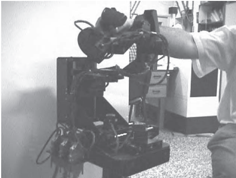
Figura 11.7. PERForce: Ejemplo de Joystick Cartesiano. (Cortesía DISAM-Universidad Politécnica de Madrid).
