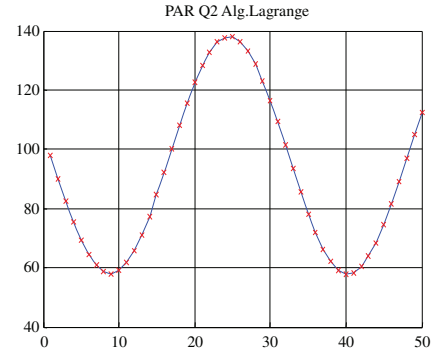
Figura 5.20. Trayectoria con sólo el segundo gdl en movimiento y pares correspondientes.
