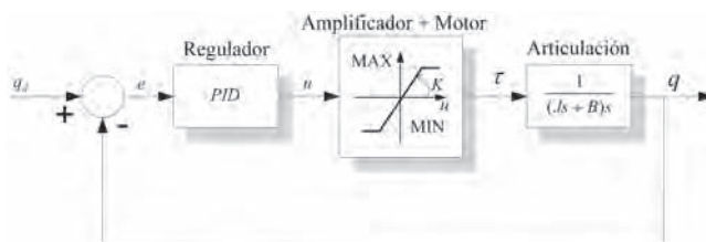
Figura 7.21. Control PID monoarticular con saturación en el amplificador.
