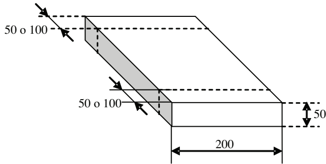
Figura 8.14. Cortes a realizar, en la tarea del Ejercicio 8.14.
