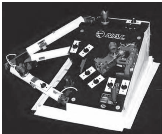
Figura 11.53. Dispositivo de experimentación Truss Structure Experiment (TSE). (Cortesía de JAXA).
