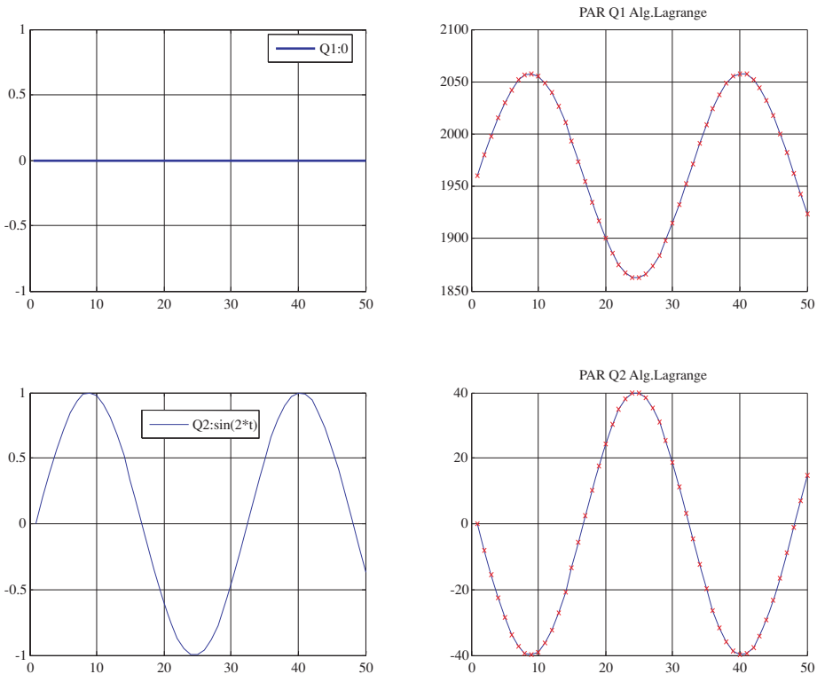
Figura 5.21. Trayectoria con sólo el segundo gdl en movimiento y primero cero.
