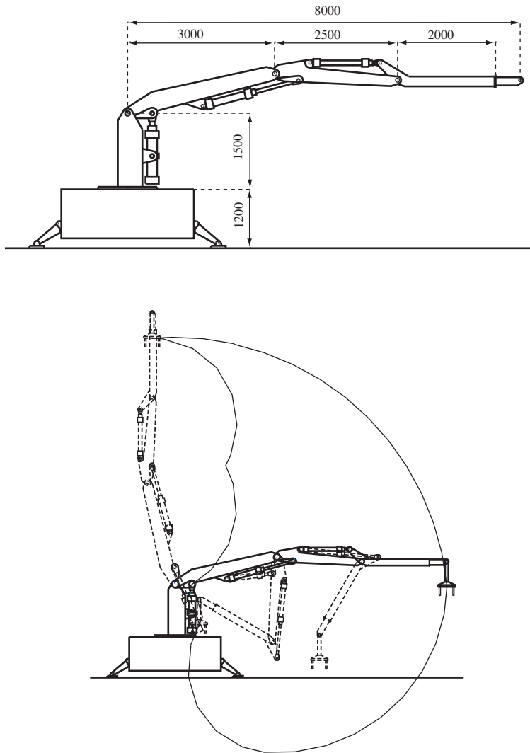
Figura 9.7. Configuración y sección del área de trabajo del robot ROCCO. (Cortesía DISAM-Universidad Politécnica de Madrid).
