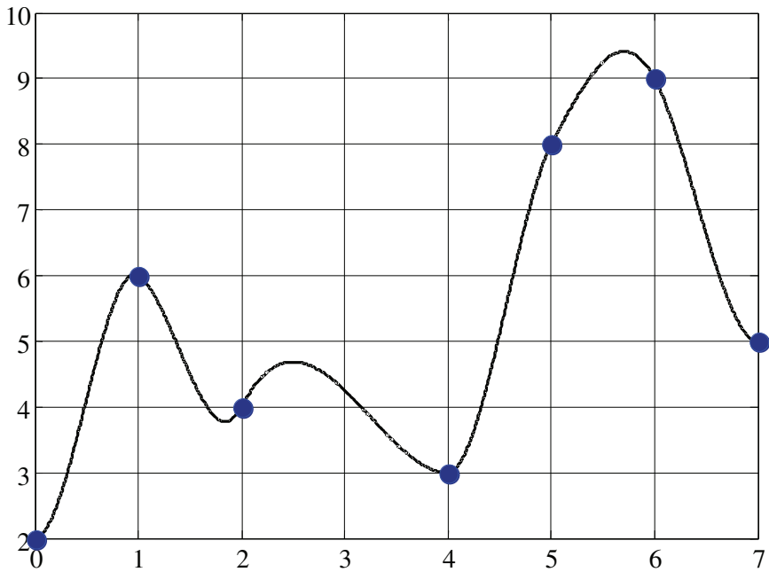
Figura 6.11. Interpolación de puntos del Ejercicio 6.2, con las velocidades de paso especificadas en el enunciado.
