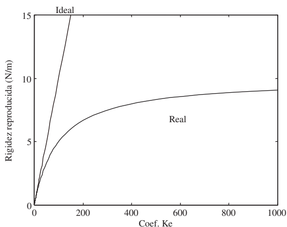
Figura 11.69. Comportamiento del bloque de reproducción de rigidez en régimen permanente para los sistemas posición-posición y fuerza-posición en función de k_e (Curva obtenida con los parámetros de la Tabla 11.11 con k_f = 0,1 ).
