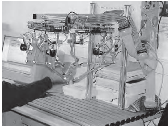
Figura 11.8. Ejemplo de joystick paralelo. (Cortesía de la Universidad Miguel Hernández).
