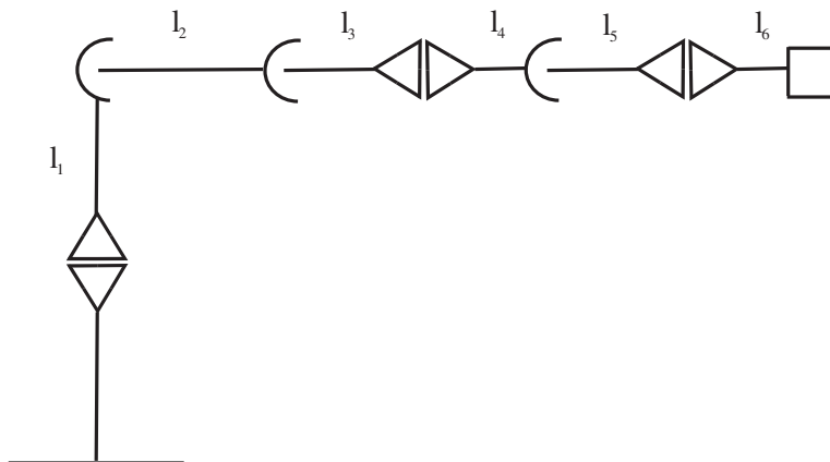
Figura 4.33. Robot de 6 GDL del Ejercicio 4.8.
