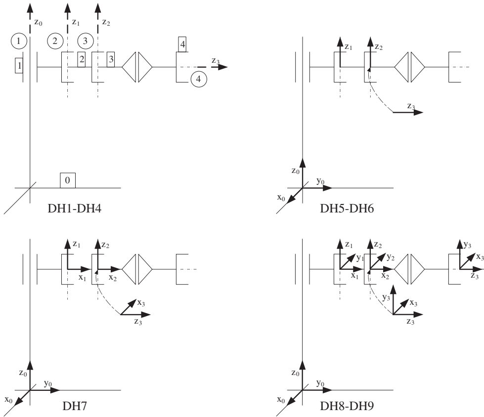
Figura 4.24. Secuencia del algoritmo de D-H para el robot del ejercicio 4.3.
