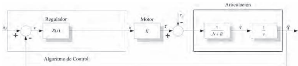
Figura 7.8. Esquema de control realimentado.
