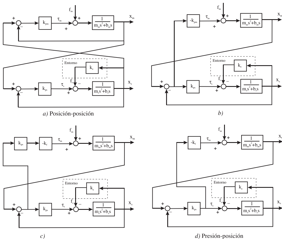
Figura 11.67. Paso mediante diagrama de bloques del esquema posición-posición al esquema presión-posición.
