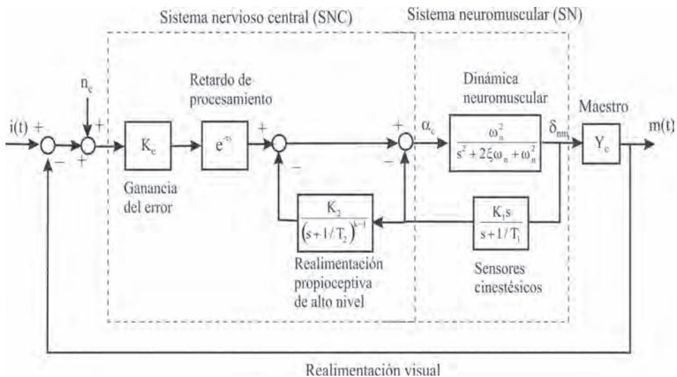
Figura 11.16. Diagrama de bloques del modelo estructural del operador para tareas de tipo compensatorio.
