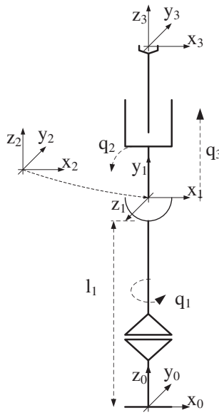
Figura 4.37. Robot esférico del Ejercicio 4.10.
