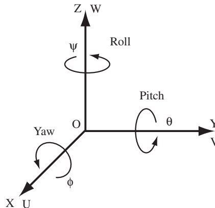
Figura 3.9. Ángulos de Euler XYZ (Yaw, Pitch y Roll).
