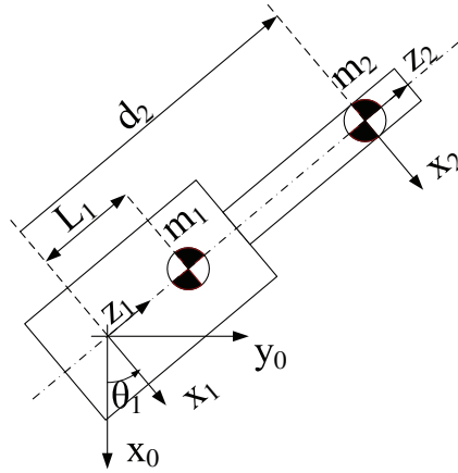
Figura 5.17. Robot polar de 2 gdl en configuración horizontal del Ejercicio 5.5.
