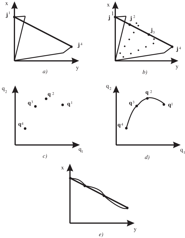
Figura 6.2. Ejemplo de las fases del control cinemático en un robot de 2 grados de libertad.
