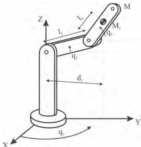
Figura 7.15. Robot articular de 3 grados de libertad.
