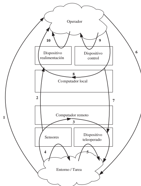
Figura 11.37. Funciones de supervisión de un operador como serie de bucles anidados [Sheridan-92].
