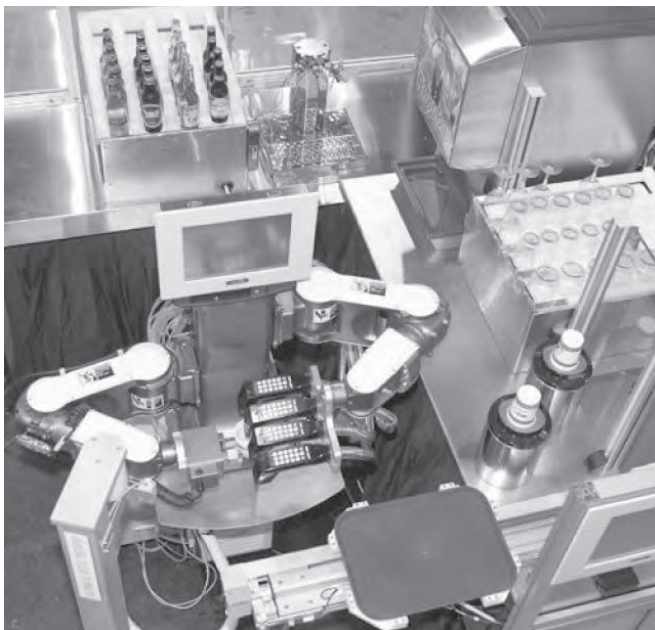
Figura 10.27. Robot Barman «Robobar». (Cortesía Motoman).
