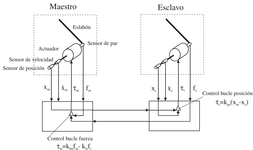
Figura 11.31. Esquema de control bilateral servo fuerza-posición.
