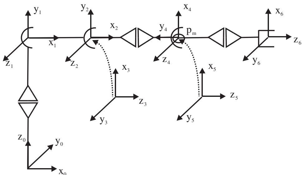
Figura 4.34. Sistemas de referencia de D-H para el robot del Ejercicio 4.8.
