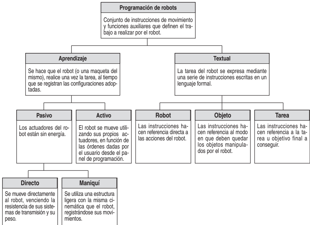
Figura 8.4. Modos de programación de Robots Manipuladores.
