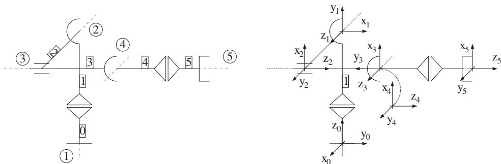
Figura 4.26. Secuencia algoritmo de DH para el robot del Ejercicio 4.4.
