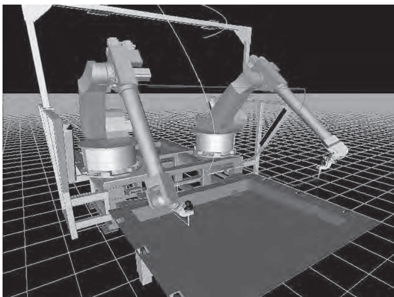
Figura 9.8. Simulador de Robots WorkSpace. (Cortesía Flow Software Technology. ROBOTNIK AUTOMATION SLL).
