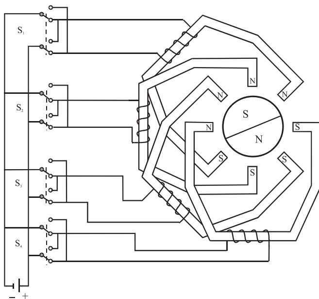
Figura 2.20. Esquema de motor paso a paso de imanes permanentes con cuatro fases.
