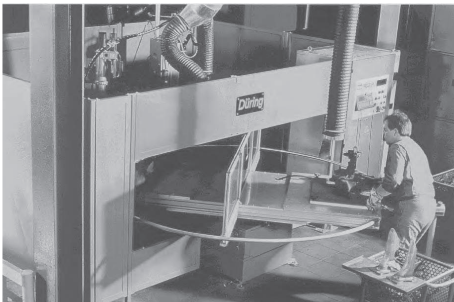
Figura 9.11. Operario utilizando una mesa giratoria para la alimentación de piezas en una célula robotizada de soldadura (Cortesía KUKA).
