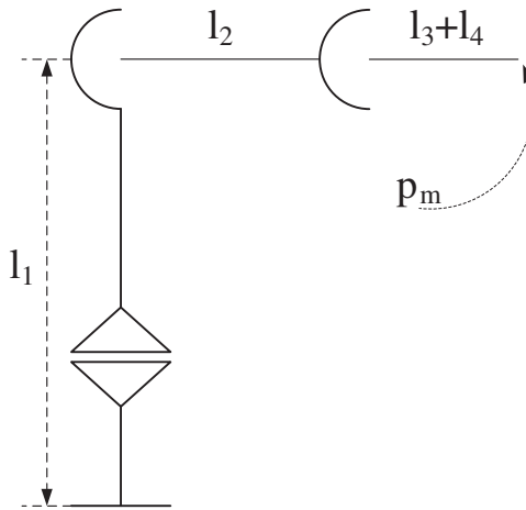
Figura 4.35. Primeros tres grados de libertad del robot del Ejercicio 4.8.
