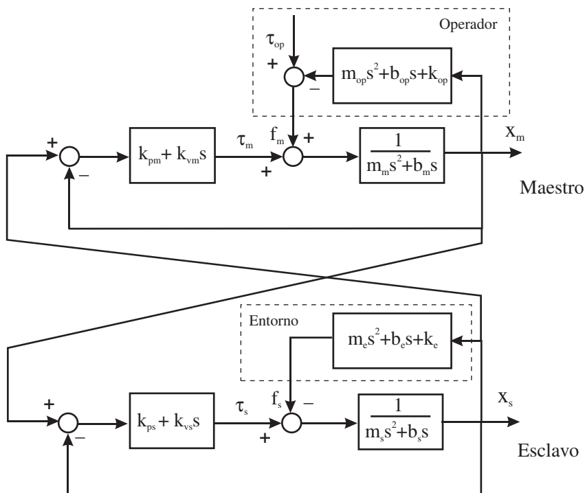
Figura 11.62. Diagrama de bloques del esquema de control bilateral posición-posición.
