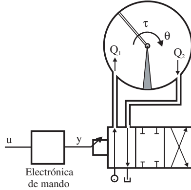
Figura 5.11. Esquema de un actuador hidráulico rotativo.
