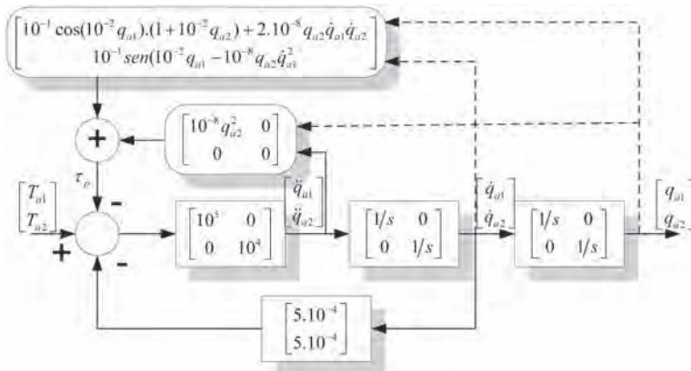
Figura 7.3. Diagrama de bloques del modelo dinámico del robot del Ejemplo 7.1.
