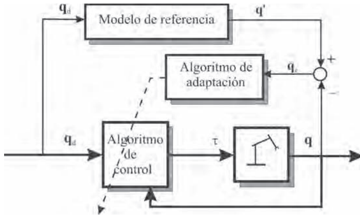
Figura 7.17. Funcionamiento de un controlador MRAC.
