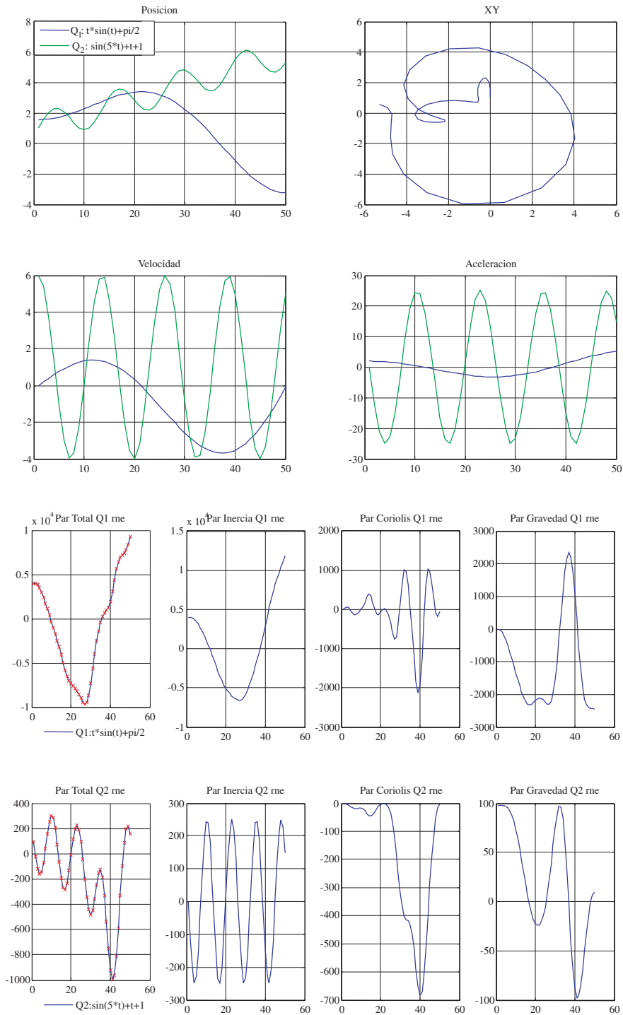
Figura 5.23. Trayectoria y Pares correspondientes a la trayectoria con los 2 gdl en movimiento obtenida con la función rne .
