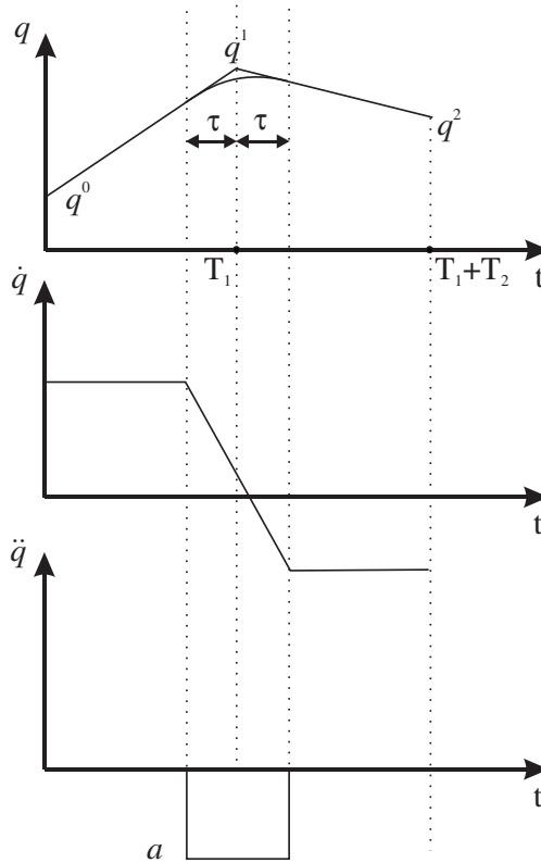
Figura 6.6. Interpolador Trapezoidal con velocidades inicial y final no nulas.
