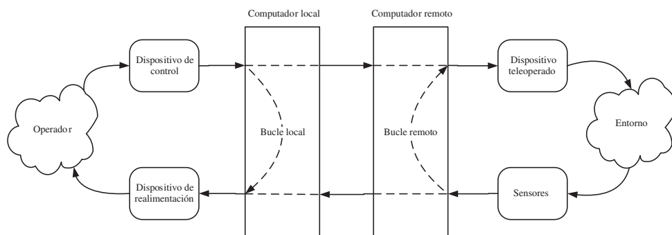
Figura 11.3. Elementos básicos de un sistema de teleoperación.
