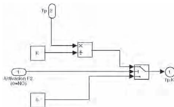
Figura 7.30. Bloque F_2(s) . Prealimentación para compensación de la perturbación.
