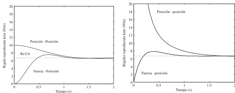
Figura 11.70. Evolución temporal de la impedancia equivalente k_{em} ( H_{pp} y H_{fp} ) para los esquemas fuerza-posición y posición-posición a) sin acción derivativa y b) con acción derivativa (Curva obtenida con los parámetros de la Tabla 11.11 y k_e = 200 N/m).
