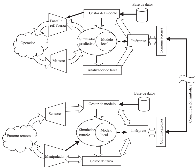
Figura 11.39. Elementos de un sistema de tele-programación.
