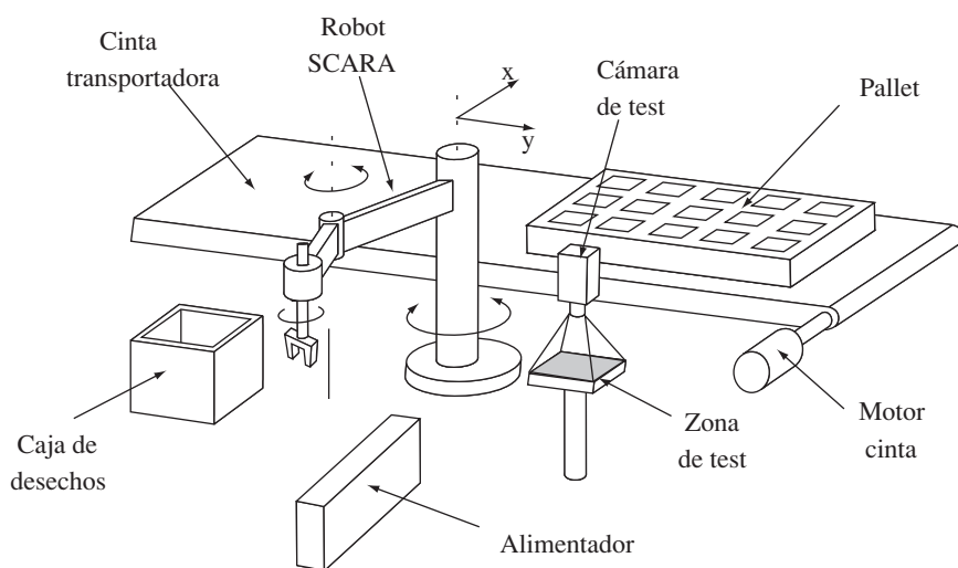
Figura 8.8. Esquema de la aplicación programada con Código-R.
