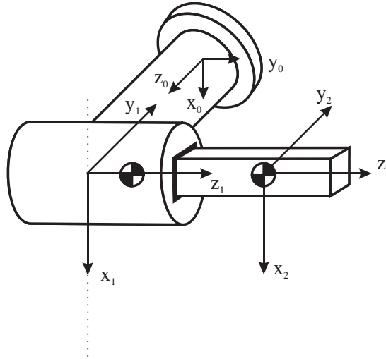
Figura 5.5. Robot polar del Ejemplo 5.1 en configuración tumbada.
