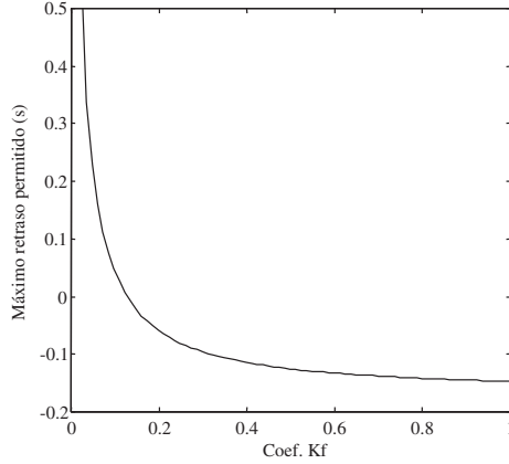
Figura 11.66. Máximo retraso permitido en un sistema fuerza-posición en función de k_f (Obtenido con los valores del sistema de la Tabla 11.11).
