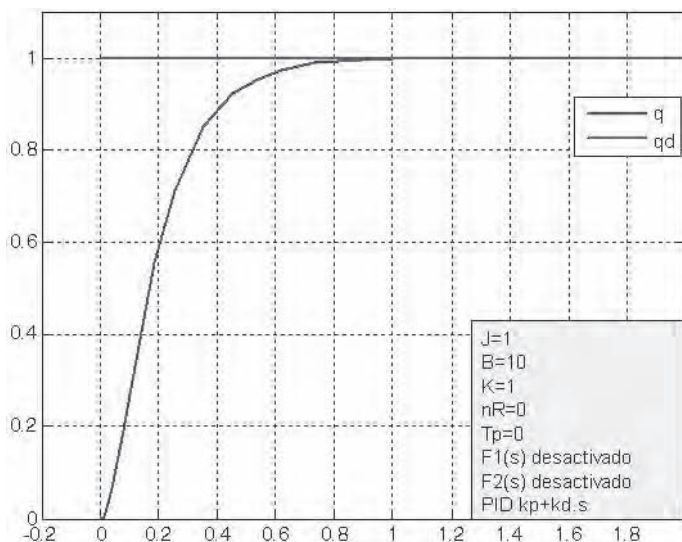
Figura 7.48. Respuesta al escalón con regulador PD ajustado.
