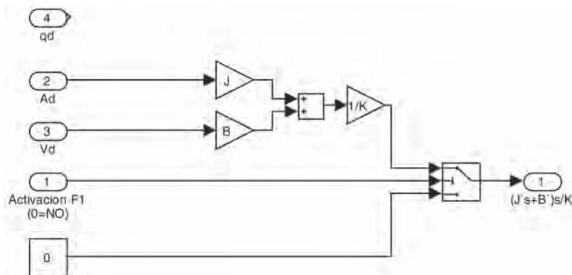
Figura 7.29. Bloque F_1(s) . Prealimentación por inversión del modelo.
