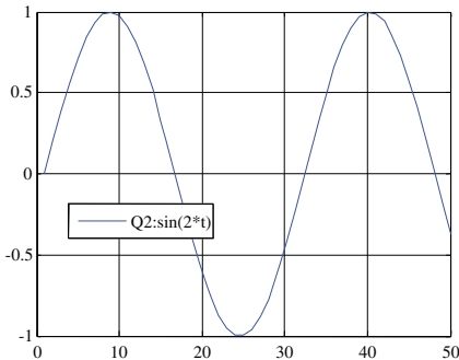
Figura 5.20. Trayectoria con sólo el segundo gdl en movimiento y pares correspondientes.
