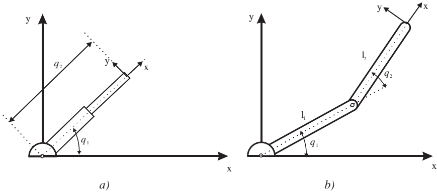
Figura 4.2. Robots planares de 2 grados de libertad.
