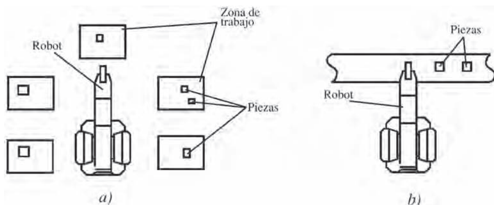
Figura 9.3. Disposición del robot en a) el centro de la célula y b) en línea.
