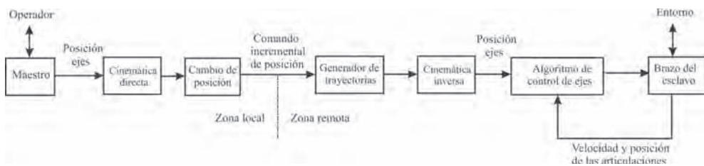
Figura 11.20. Esquema general de control unilateral integrado.
