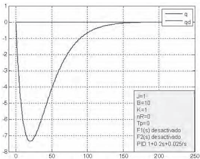
Figura 7.44. Compensación del par perturbador mediante una acción integral media.
