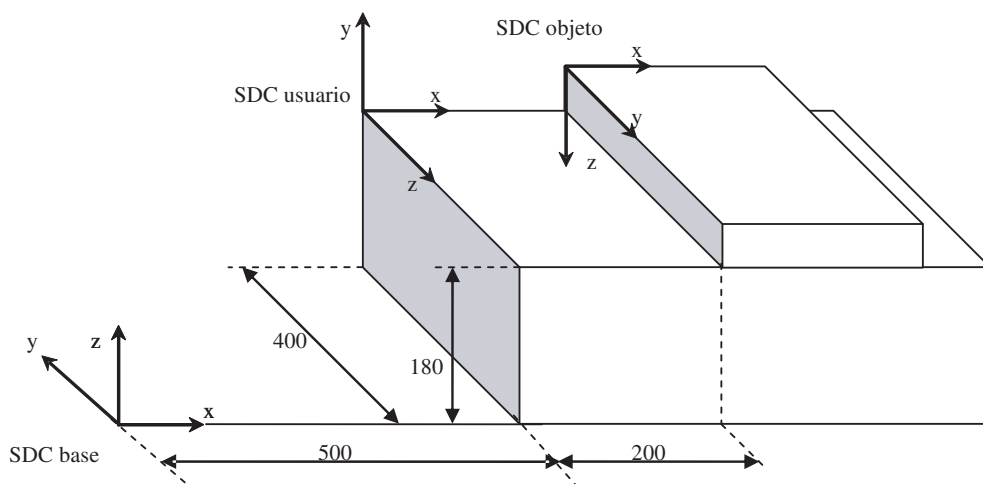
Figura 8.15. Disposición del entorno de trabajo del Ejercicio 8.14.
