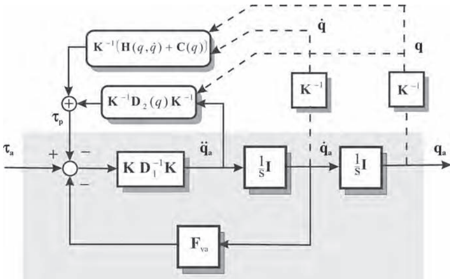
Figura 7.1. Diagrama de bloques que representa el comportamiento dinámico de una articulación.
