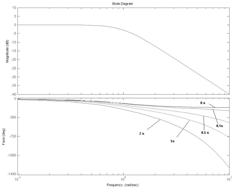
Figura 11.24. Diagrama de Bode de un sistema de segundo orden ( \omega_n = 1 rad/s y \zeta = 0,7 ) realimentado con distintos retardos.
