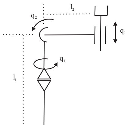
Figura 4.30. Robot del Ejercicio 4.7.
