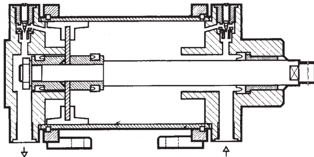
Figura 2.13. Esquema de cilindro neumático de doble efecto. (Cortesía de FESTO).
