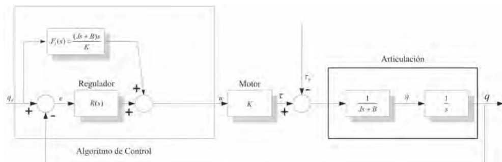
Figura 7.11. Control pre-alimentado + realimentado.
