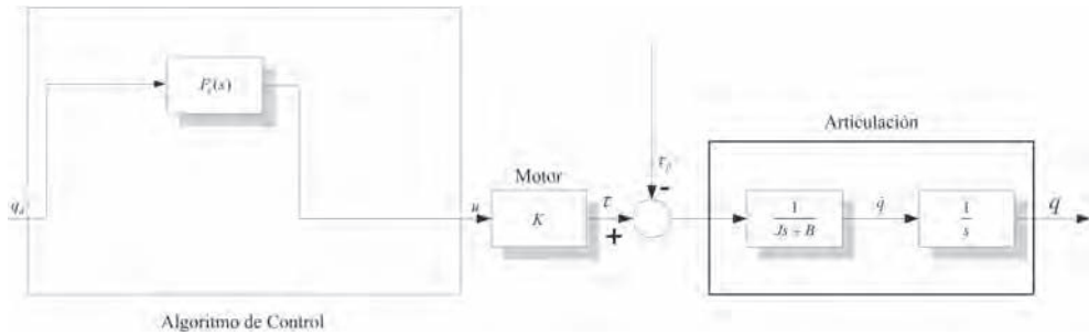
Figura 7.7. Esquema de control por prealimentación. (Feed-forward).
