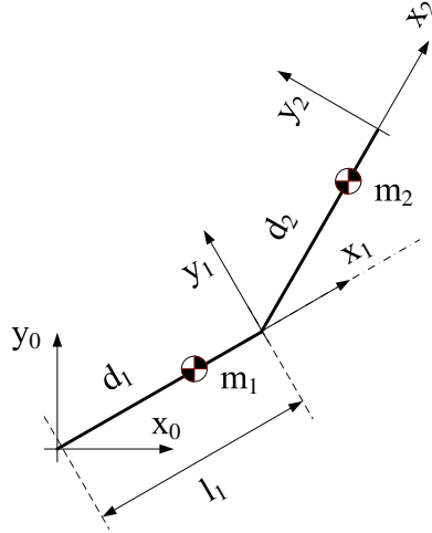
Figura 5.24. Robot planar de 2 grados de libertad del Ejercicio 5.2.
