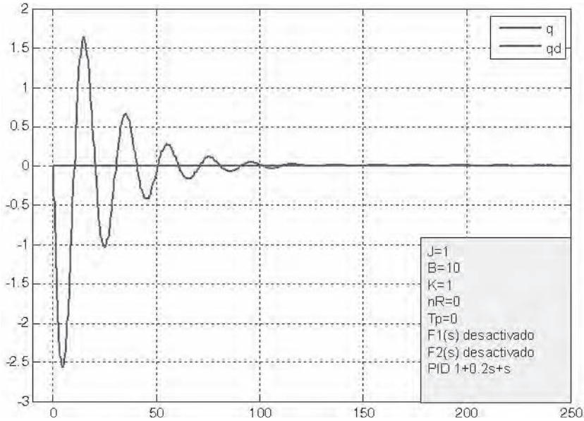
Figura 7.45. Compensación del par perturbador mediante una acción integral alta.
