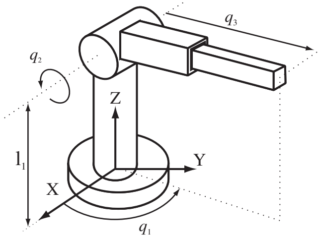
Figura 4.11. Robot polar de 3 GDL.
