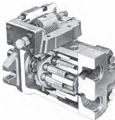
Figura 2.15. Motor de pistones axiales. (Cortesía FESTO).
