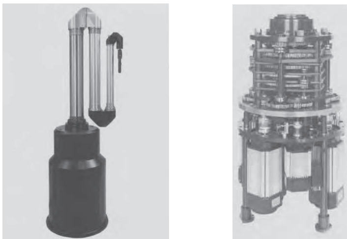
Figura 2.8. Telemanipulador TELBOT junto con la caja de transmisión por engranajes situada en su base. (Cortesía de Wälischmiller GmbH).
