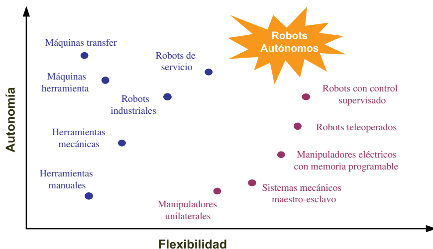
Figura 11.6. Evolución de la robótica y la teleoperación en cuanto a flexibilidad y autonomía.
