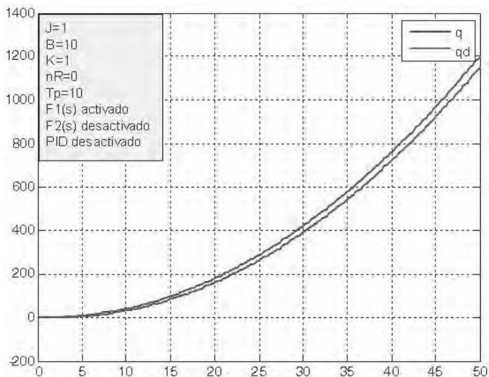
Figura 7.38. Trayectoria deseada q_d y real q con control FF y perturbación T_p = 10 .
