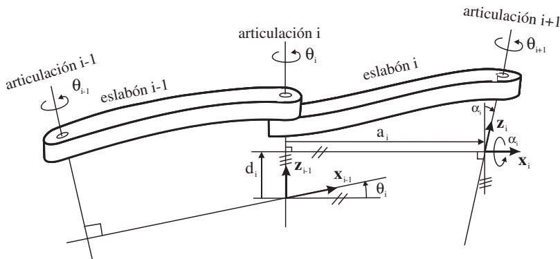
Figura 4.5. Parámetros de D-H para un eslabón giratorio.
