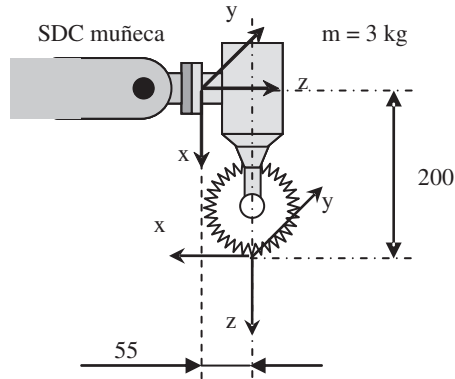
Figura 8.13. Detalle herramienta robot Ejercicio 8.14.
