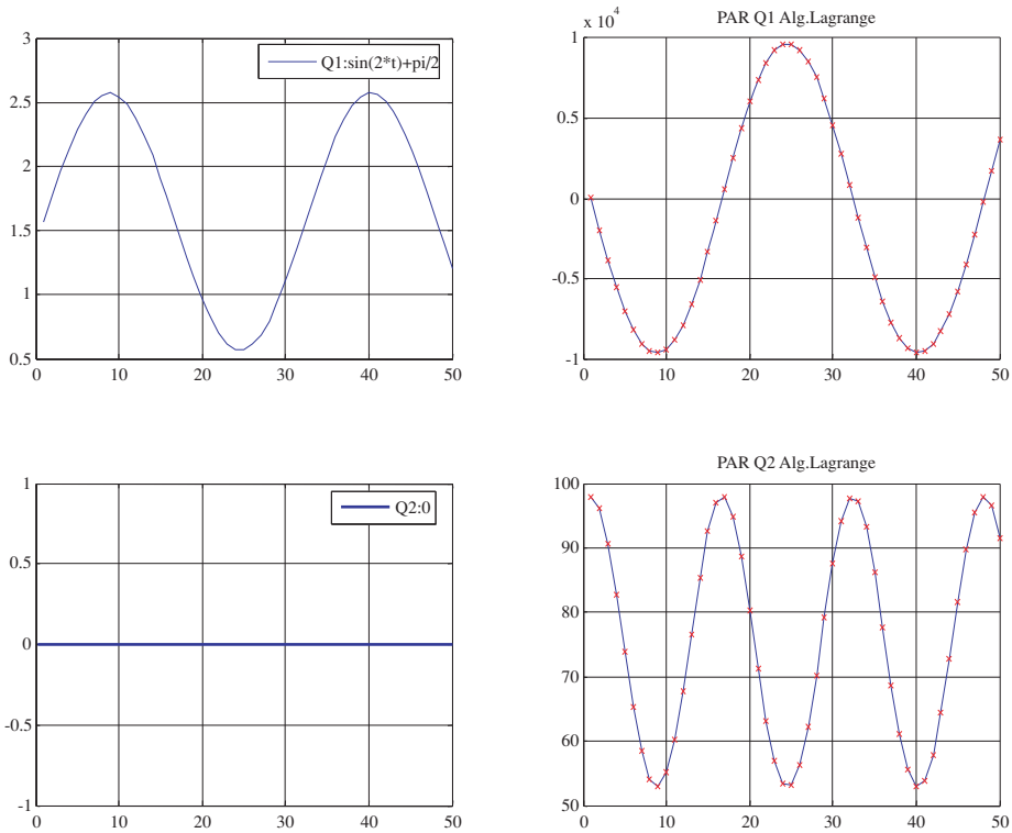
Figura 5.19. Trayectoria con sólo el primer gdl en movimiento y segundo en cero.
