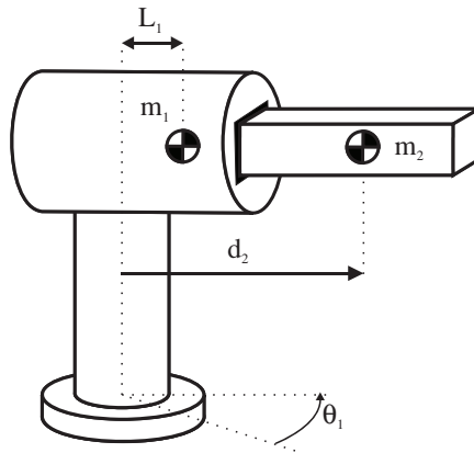
Figura 5.2. Robot polar de 2 grados de libertad del Ejemplo 5.1.
