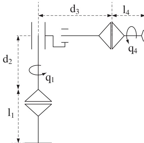
Figura 4.36. Robot cilíndrico del Ejercicio 4.9.
