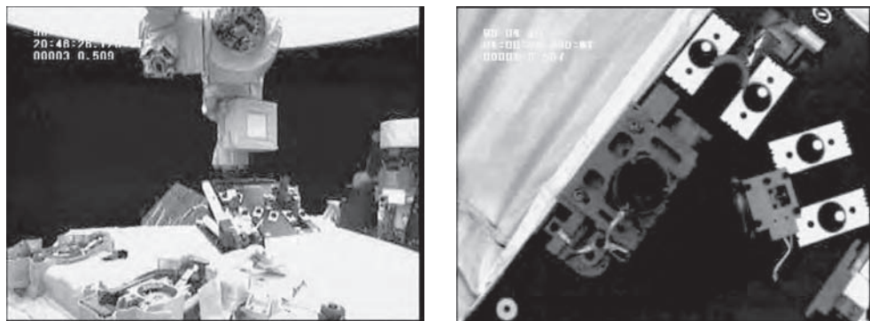
Figura 11.48. Ejemplo de imágenes proporcionadas por la cámara en la base (izquierda) y en el extremo del robot (derecha). (Cortesía de JAXA).
