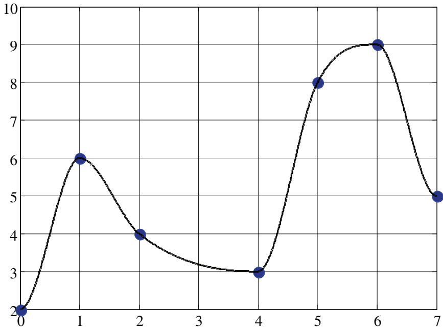
Figura 6.10. Interpolación de puntos del Ejercicio 6.2 con las velocidades de paso definidas según [6.6].
