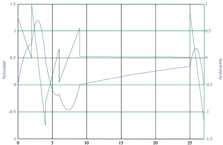
Figura 6.9. Evolución de la velocidad y aceleración de la trayectoria del Ejercicio 6.1.
