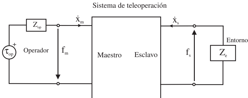
Figura 11.35. Esquema de teoría de cuadripolo aplicada a un sistema con control bilateral.
