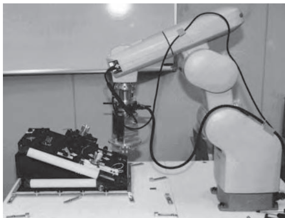
Figura 11.52. Réplica del sistema teleoperado con robot industrial que imita los movimientos del robot a bordo del satélite.
