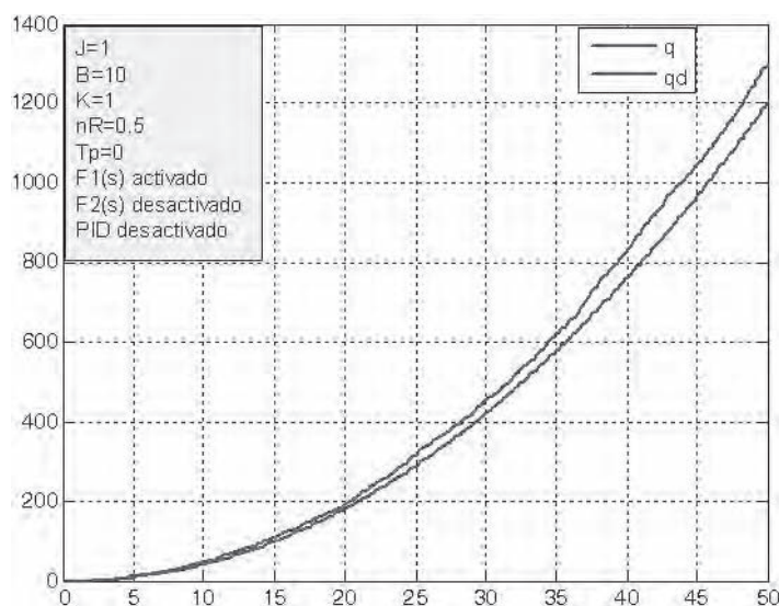
Figura 7.39. Trayectoria deseada q_d y real q con control FF y dinámica mal modelada ( nR = 0.5 ).
