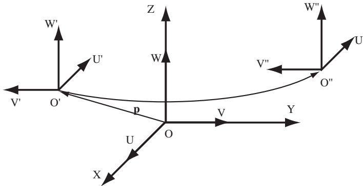
Figura 3.15. Distintos sistemas finales según el orden de las transformaciones.
