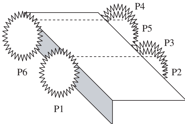
Figura 8.16. Puntos de corte del Ejercicio 8.2.
