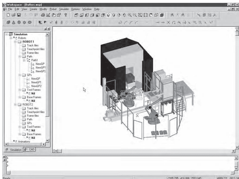
Figura 9.2. Definición del lay-out de la célula mediante simulador. (Cortesía Flow Software Technology-ROBOTNIK AUTOMATION SLL).
