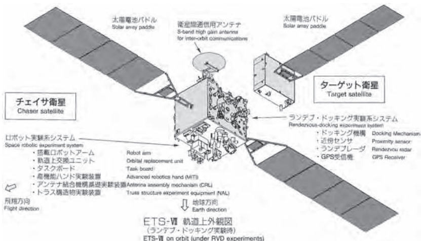
Figura 11.45. Imagen artística del ETS-VII. (Cortesía de JAXA).
