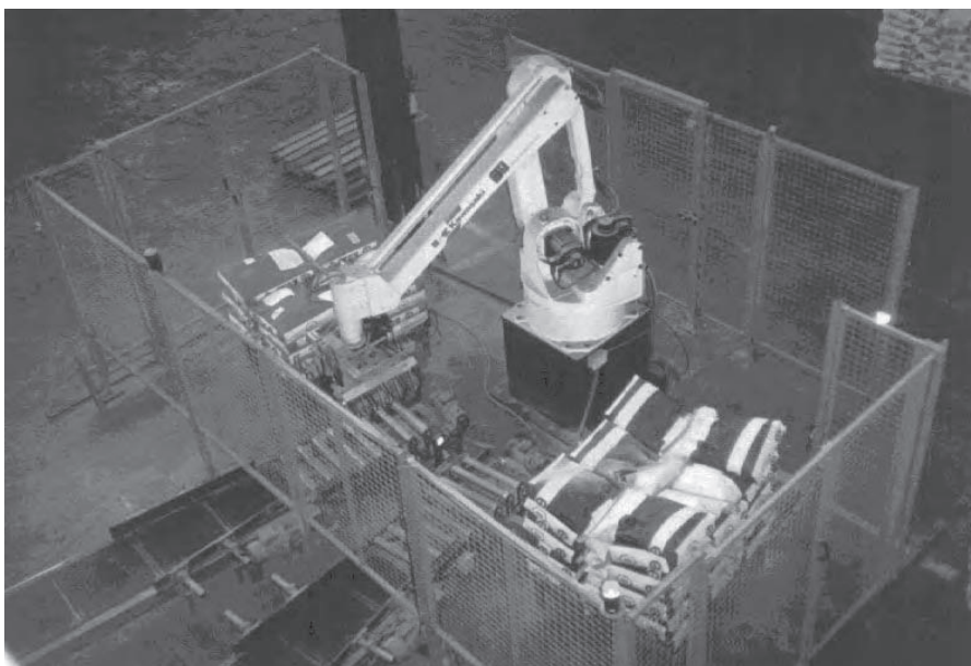
Figura 9.10. Célula robotizada de paletizado con vallas de protección para impedir el acceso. (Cortesía de INSER Robótica).
