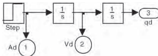
Figura 7.34. Generador de trayectoria escalón de aceleración.
