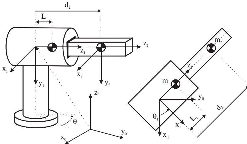
Figura 5.6. Configuración y Sistemas de referencia del robot polar del Ejemplo 5.2.
