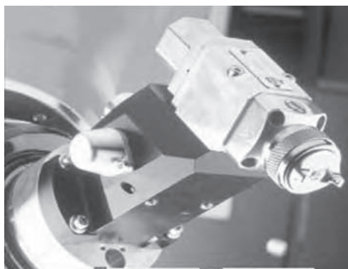
Figura 2.32. Pistola de pulverización neumática de pintura. (Cortesía de ABB).
