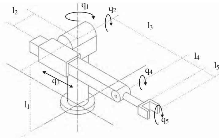
Figura 4.25. Robot del Ejercicio 4.4.
