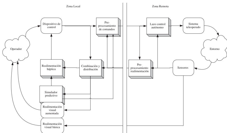
Figura 11.5. Arquitectura genérica de un sistema de teleoperación.
