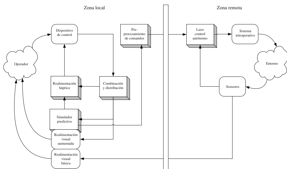
Figura 11.38. Arquitectura de tele-programación.
