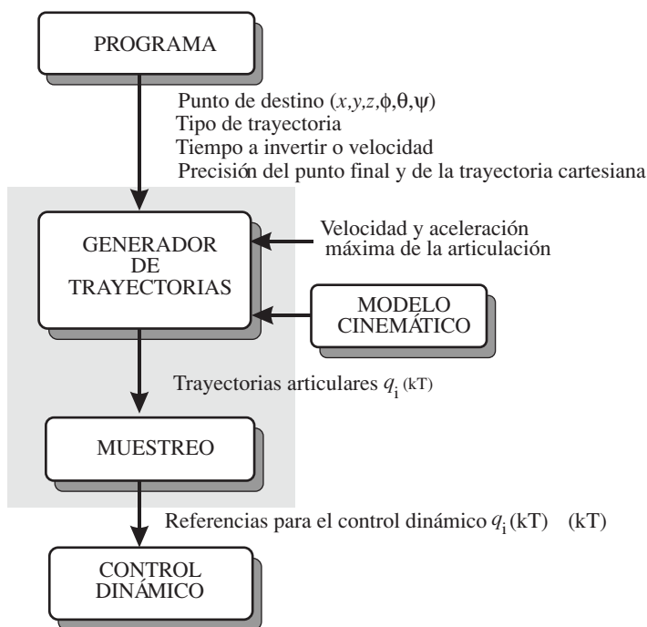
Figura 6.1. Funcionamiento del control cinemático (sombreado).
