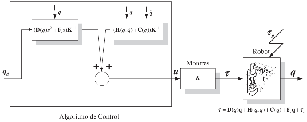
Figura 7.13. Desacoplamiento por inversión del modelo.
