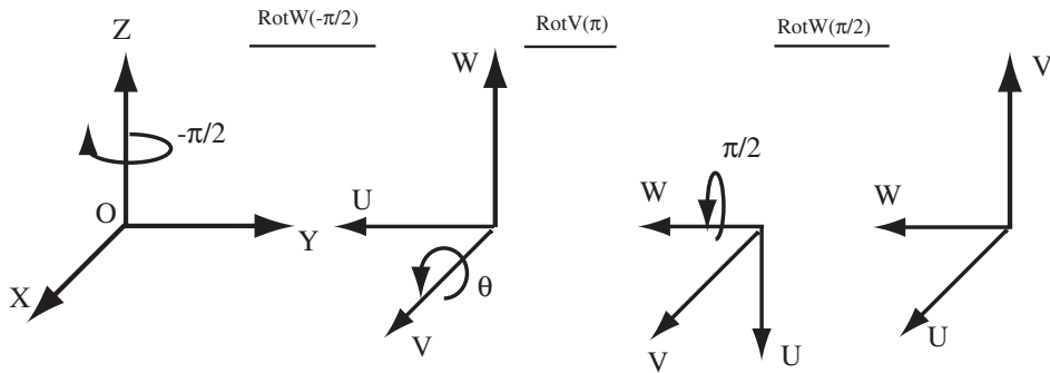
Figura 3.23. Transformaciones Ejercicio 3.5.
