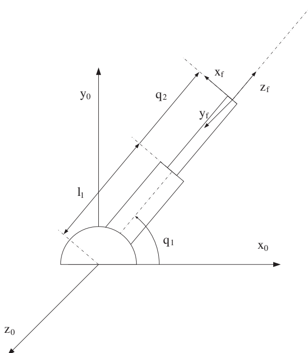
Figura 4.18. Robot Ejercicio 4.1.
