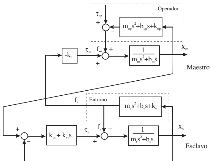
Figura 11.34. Diagrama de bloques del esquema de control bilateral fuerza-posición.
