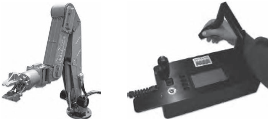
Figura 11.2. Sistema de telemanipulación TITAN 4. Manipulador esclavo y manipulador maestro. (Cortesía de Schilling Robotics Inc.).
