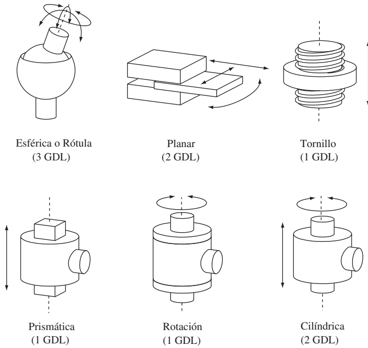
Figura 2.2. Los seis pares inferiores de Reuleaux.
