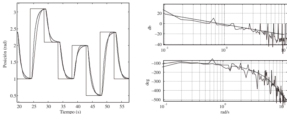
Figura 11.19. Comparación temporal y frecuencial entre la respuesta experimental (claro) y la respuesta del modelo de cross-over (oscuro) para un experimento de movimiento discreto utilizando un dispositivo de entrada de un grado de libertad.
