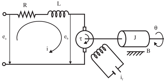
Figura 5.8. Esquema de funcionamiento de un motor de corriente continua controlado por inducido.
