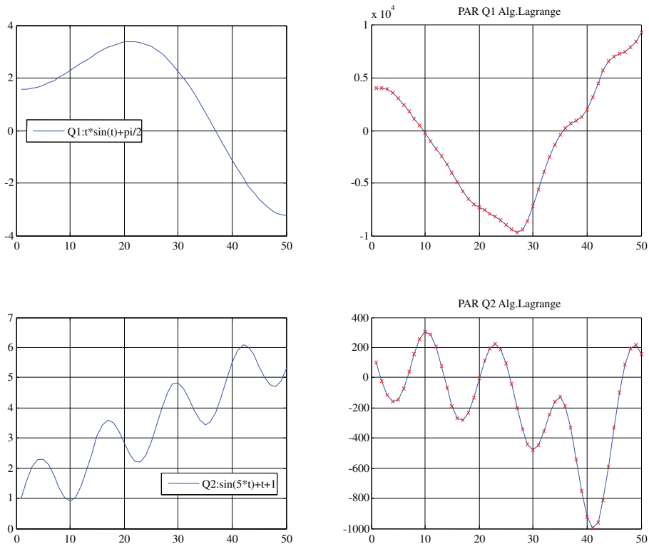
Figura 5.22. Trayectoria con 2 gdl en movimiento y pares correspondientes.
