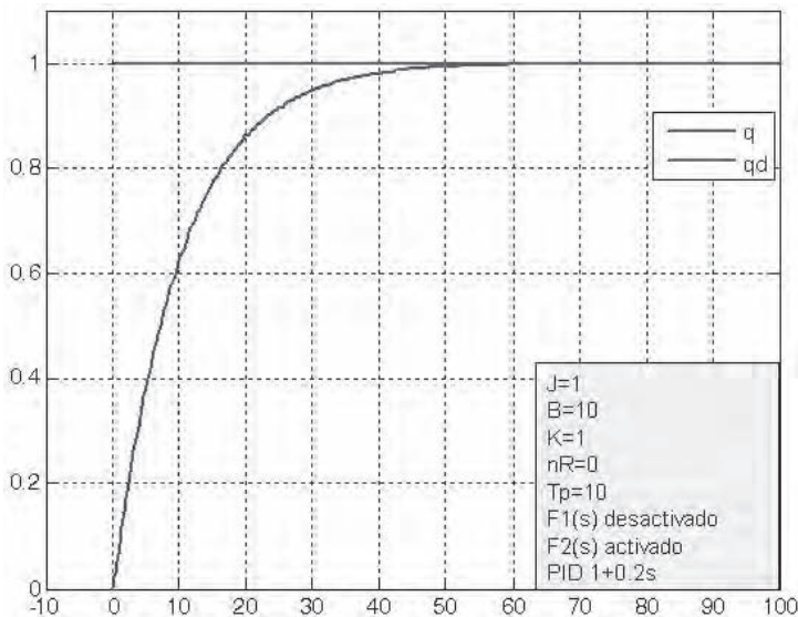
Figura 7.47. Trayectoria deseada q_d y real q ante entrada escalón y perturbación T_p de 10 unidades con control PD-G.
