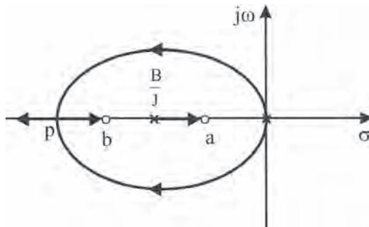
Figura 7.19. Lugar de las raíces de una articulación con control PID.
