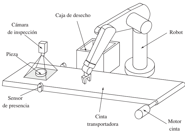
Figura 8.10. Célula robotizada de inspección para ejemplo de programación RAPID.
