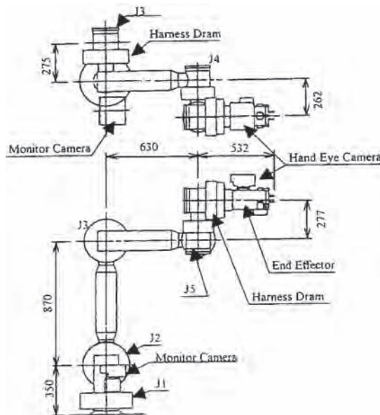
Figura 11.47. Configuración del robot a bordo del satélite ETS-VII. (Cortesía de JAXA).
