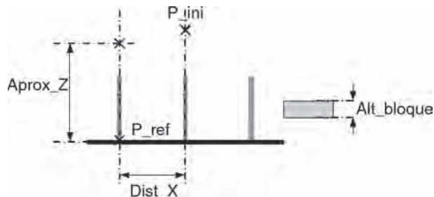
Figura 8.12. Dimensiones del tablero de las Torres de Hanoi.
