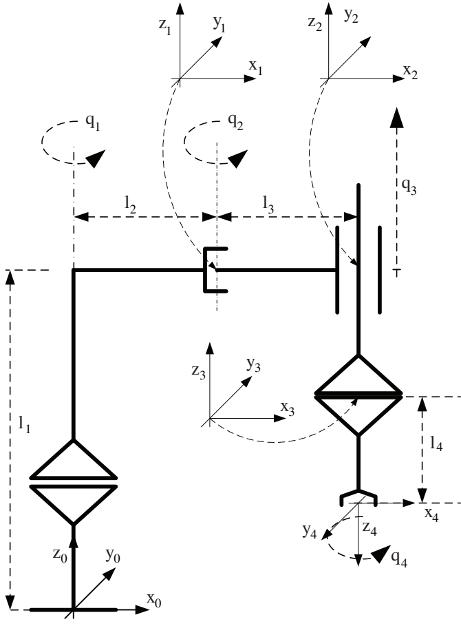
Figura 4.15. Robot Scara Ejemplo 4.4.
