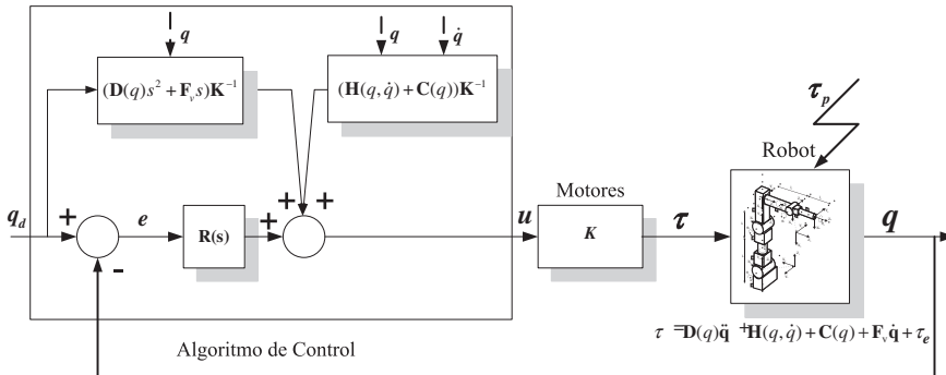
Figura 7.14. Esquema de algoritmo de control basado en PID y prealimentación sobre el sistema desacoplado.
