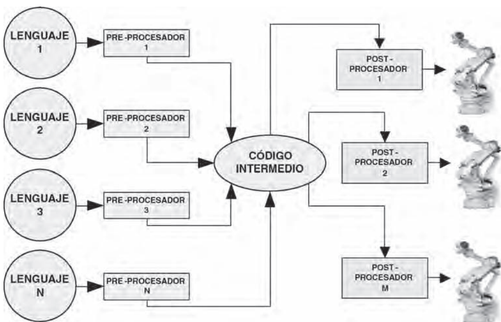
Figura 8.7. Uso de un código intermedio como interfase entre lenguajes genéricos y robots.
