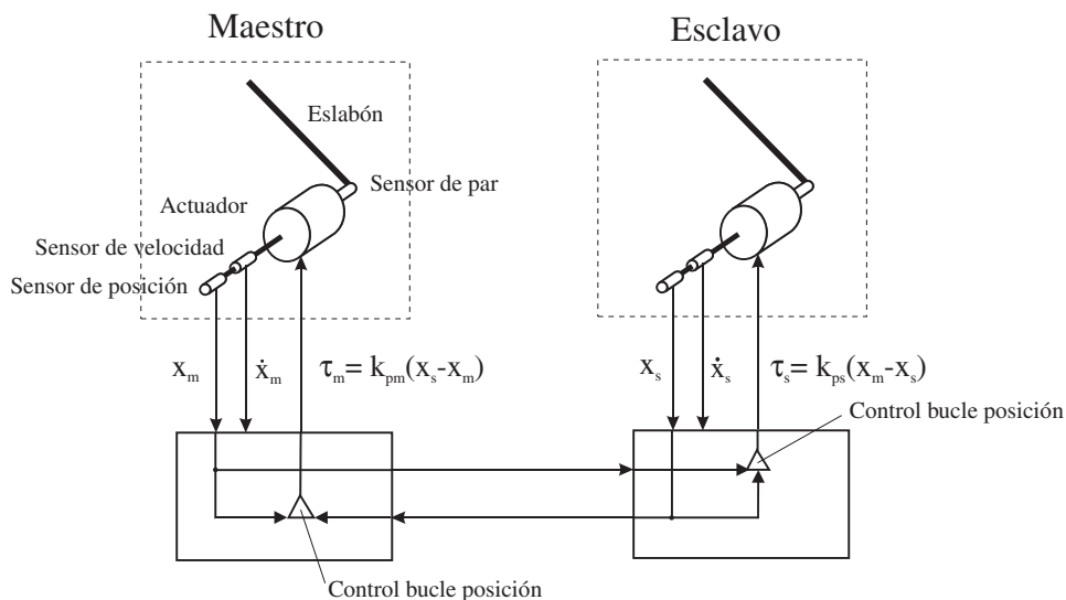
Figura 11.29. Esquema de control bilateral posición-posición.
