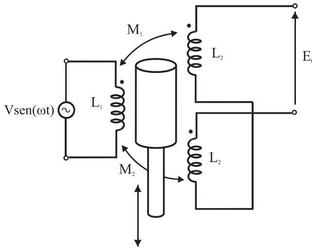
Figura 2.27. Esquema de funcionamiento de un LVDT.
