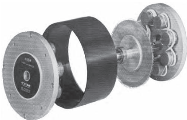
Figura 2.19. Motor de Corriente Continua de imanes permanentes y rotor serigrafiado.
