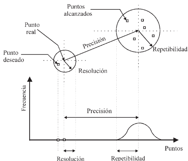
Figura 9.9. Visualización de los conceptos de resolución, precisión y repetibilidad.
