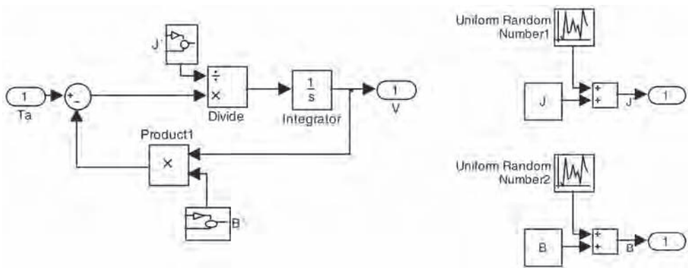
Figura 7.32. Subsistema que implementa el modelo de la articulación y detalle de los subsistemas ( J' ) y B' .
