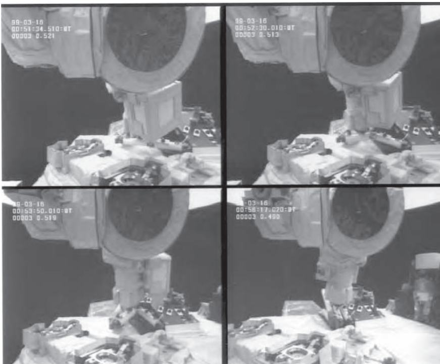
Figura 11.58. Secuencia de plegado de la estructura sobre el TSE. (Cortesía de JAXA).
