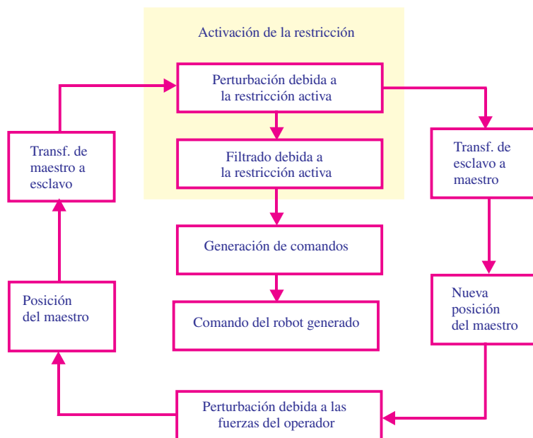
Figura 11.41. Flujo de información en la implementación de un sistema de tele-programación con restricciones virtuales.
