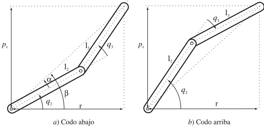
Figura 4.10. Elementos 2 y 3 del robot de la Figura 4.9 contenidos en un plano y en a) configuración codo abajo y b) configuración codo arriba.
