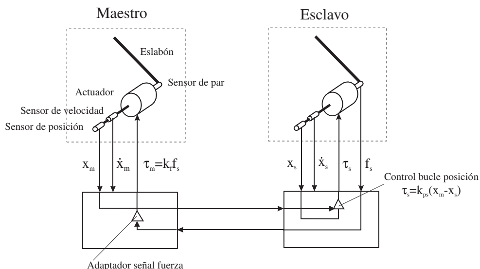
Figura 11.30. Esquema de control bilateral fuerza-posición.
