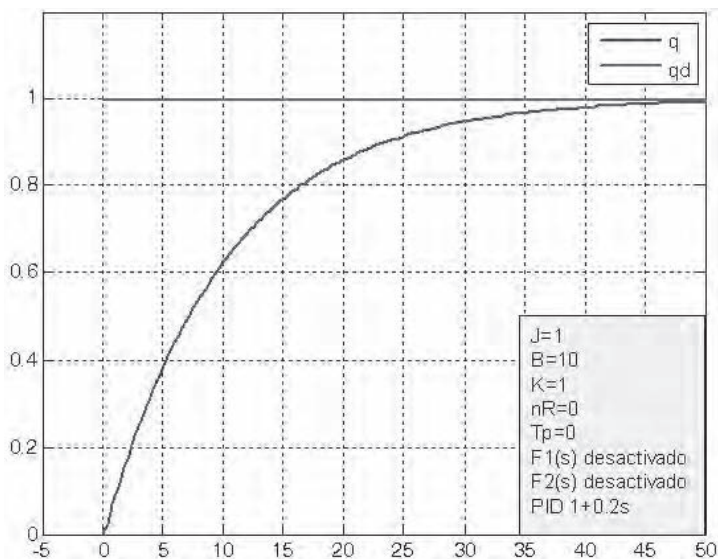
Figura 7.40. Trayectoria deseada q_d y real q ante entrada en escalón con control PD.
