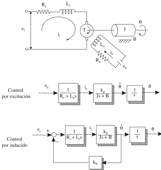
Figura 2.18. Motor DC- Esquema y funciones de transferencia.
