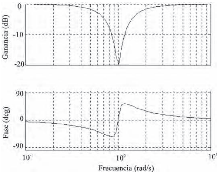
Figura 7.27. Diagrama de Bode de un filtro de muesca.
