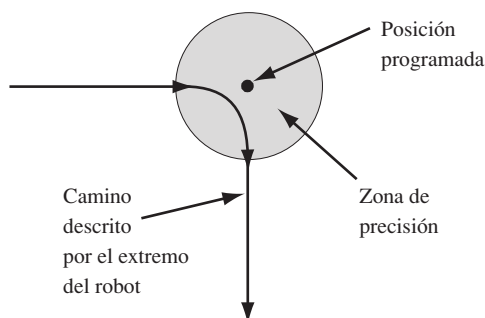
Figura 8.6. Funcionamiento de un punto de paso ( via point ).
