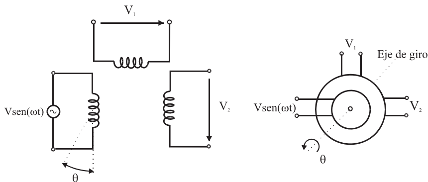
Figura 2.25. Esquema de funcionamiento de un resolver.
