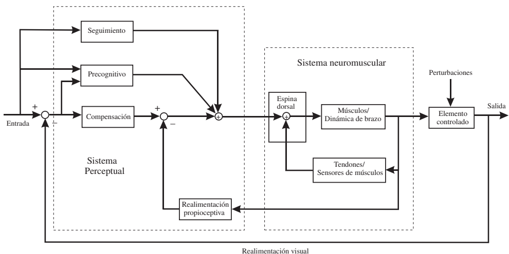
Figura 11.15. Elementos principales en el control manual por un operador.
