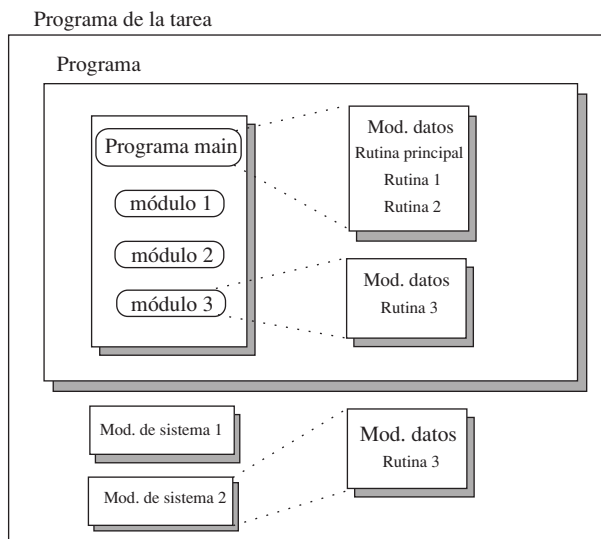
Figura 8.9. Estructura de un programa RAPID.
