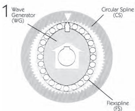
Figura 2.10. Esquema Reductor Armónico. (Cortesía Harmonic Drive).
