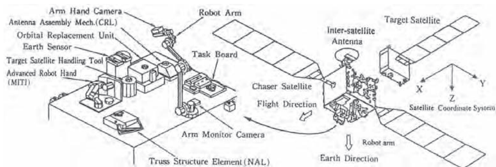
Figura 11.46. Detalle de los equipos situados sobre una de las caras exteriores del satélite ETS-VII (Cortesía de JAXA).
