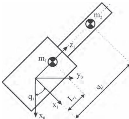
Figura 7.2. Eslabones del robot del Ejemplo 7.1.
