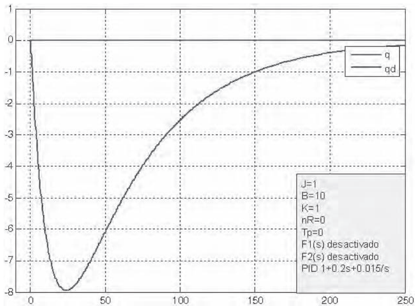
Figura 7.43. Compensación del par perturbador mediante una acción integral baja.
