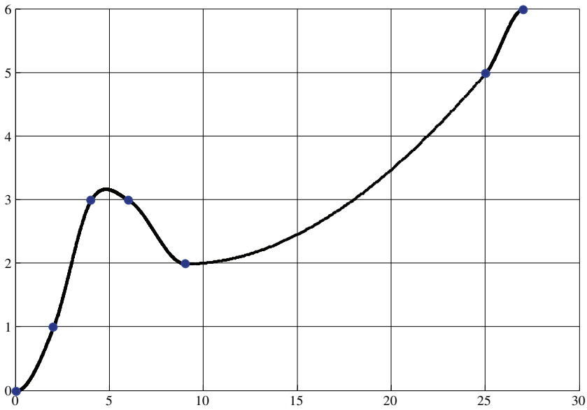
Figura 6.8. Interpolación de los puntos del Ejercicio 6.1 mediante spline cúbico.
