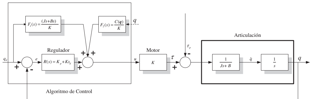
Figura 7.12. Control PD + FF + G.
