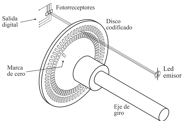
Figura 2.22. Disposición de un codificador óptico (encoder) incremental.
