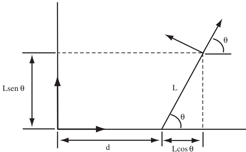
Figura 3.26. Resolución por consideraciones geométricas del Ejercicio 3.8.
