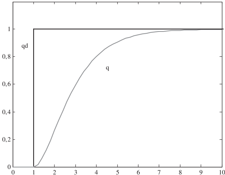
Figura 7.9. Respuesta de la articulación ante q_d escalón con R(s) no nulo.
