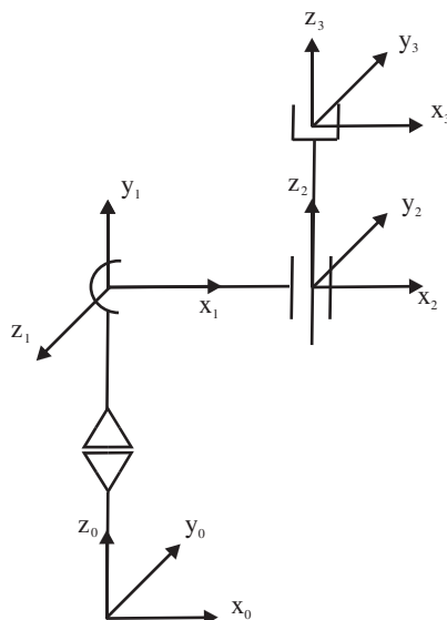
Figura 4.32. Sistemas de D-H para el robot de Ejercicio 4.7.
