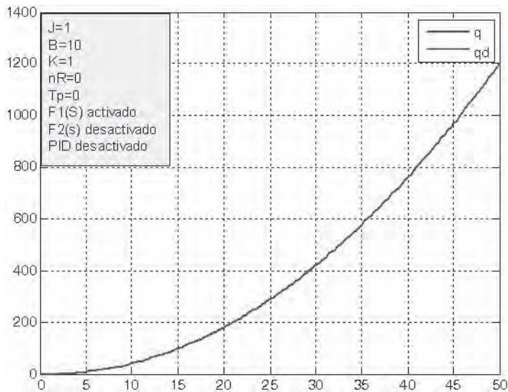
Figura 7.37. Trayectoria deseada q_d y real q (coincidentes) con control FF sin perturbación.
