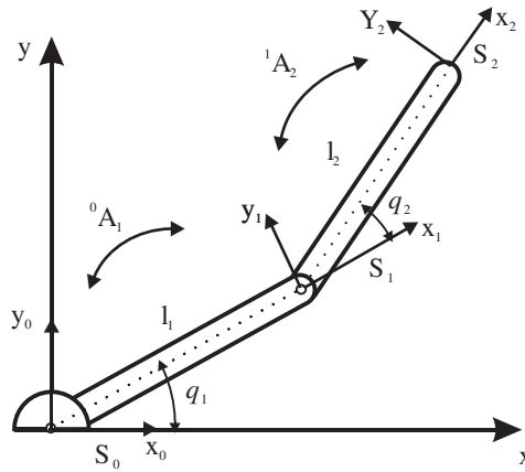
Figura 4.4. Asociación de sistemas de referencia a cada eslabón del robot.
