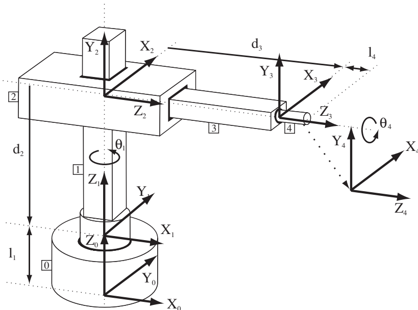
Figura 4.6. Robot cilíndrico del Ejemplo 4.2.
