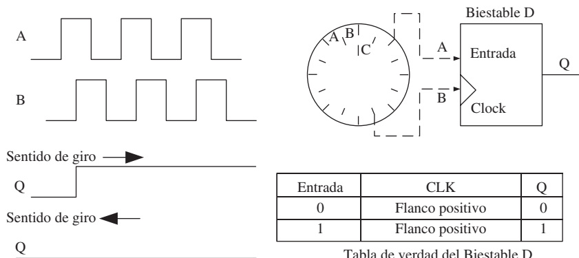
Figura 2.23. Salidas A y B de un encoder y valor (Q) del biestable D, según sentido de giro.
