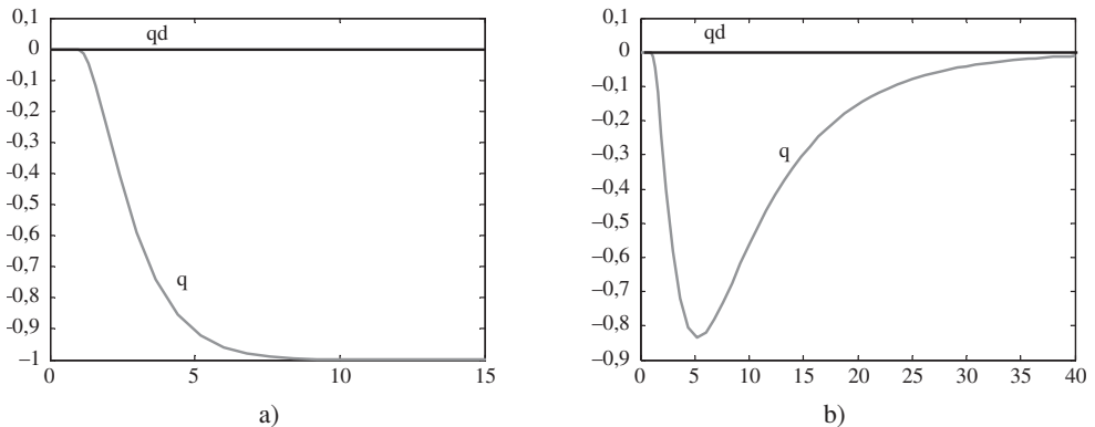
Figura 7.10. Respuesta a perturbación t_p escalón con (a) Regulador P, (b) Regulador PI.
