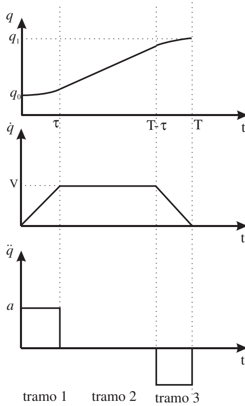
Figura 6.5. Interpolador Trapezoidal.
