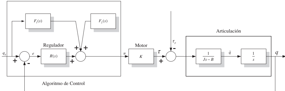
Figura 7.6. Esquema general de control monoarticular.
