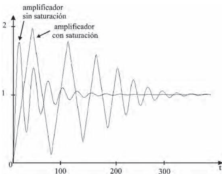
Figura 7.22. Comparación de respuesta con y sin saturación.
