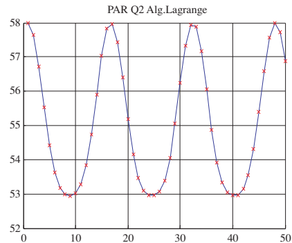
Figura 5.18. Trayectoria con sólo el primer gdl en movimiento y pares correspondientes.
