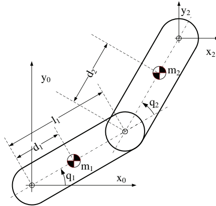
Figura 5.15. Robot planar de 2 grados de libertad del Ejercicio 5.2.
