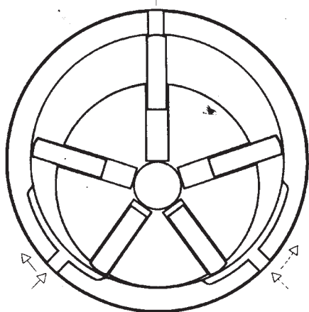
Figura 2.14. Motor de paletas. (Cortesía FESTO).
