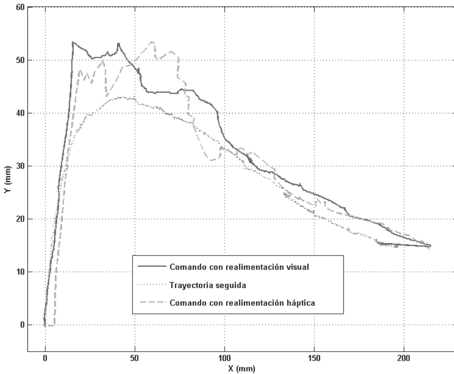
Figura 11.60. Comparación entre las trayectorias del experimento de plegado utilizando únicamente realimentación visual o realimentación de fuerzas para guiar al operador.
