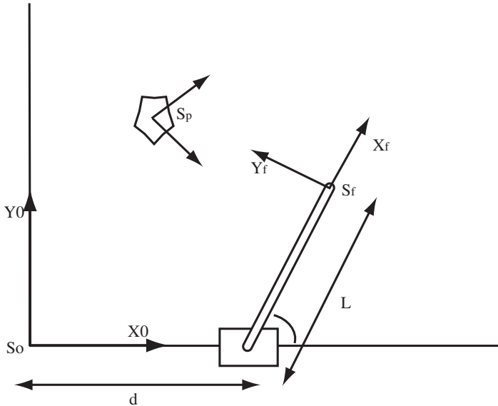
Figura 3.25. Figura Ejercicio 3.8.
