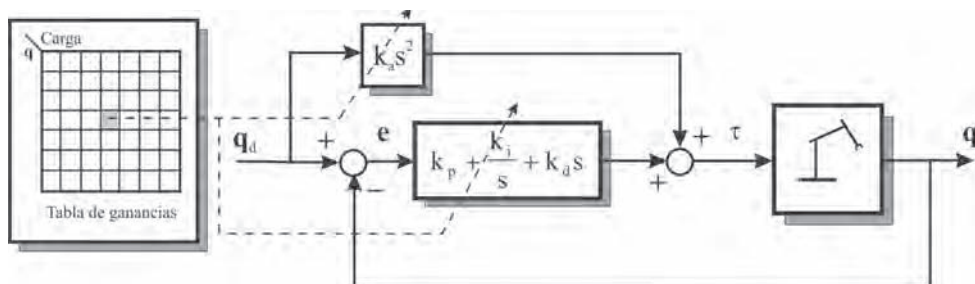
Figura 7.16. Control monoarticular con planificación de ganancias.
