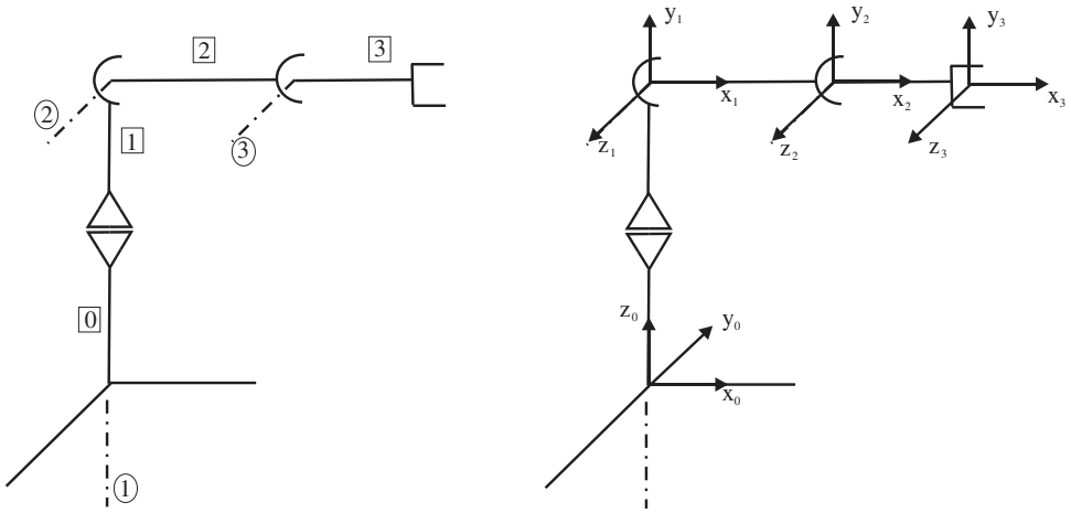
Figura 4.29. Secuencia de D-H para el robot del Ejercicio 4.6.
