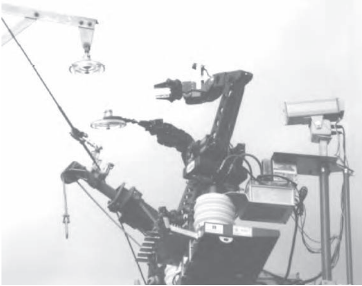
Figura 1.12. Sistema ROBTET para reparación de líneas eléctricas, con robots de accionamiento hidráulico (Cortesía DISAM - Universidad Politécnica de Madrid).
