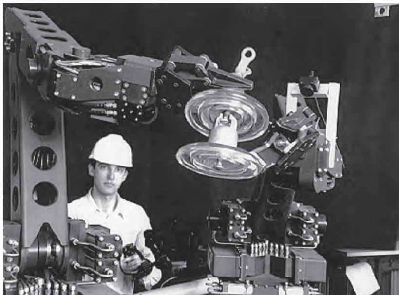
Figura 1.5. Sistema de telemanipulación bilateral.
