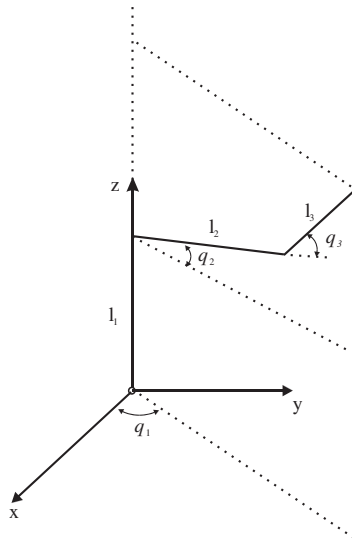
Figura 4.20. Figura Ejercicio 4.2.
