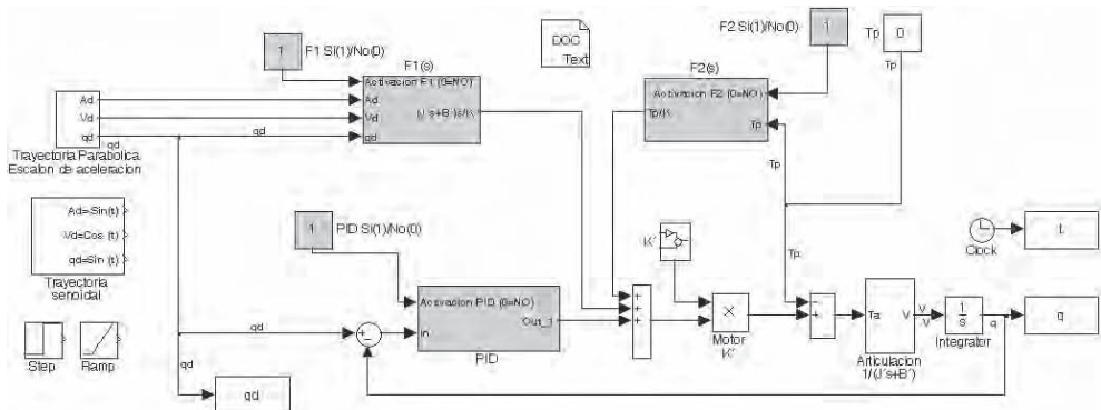
Figura 7.36. Esquema de control usando solo FF ( F_1(s) ), sin par perturbador.
