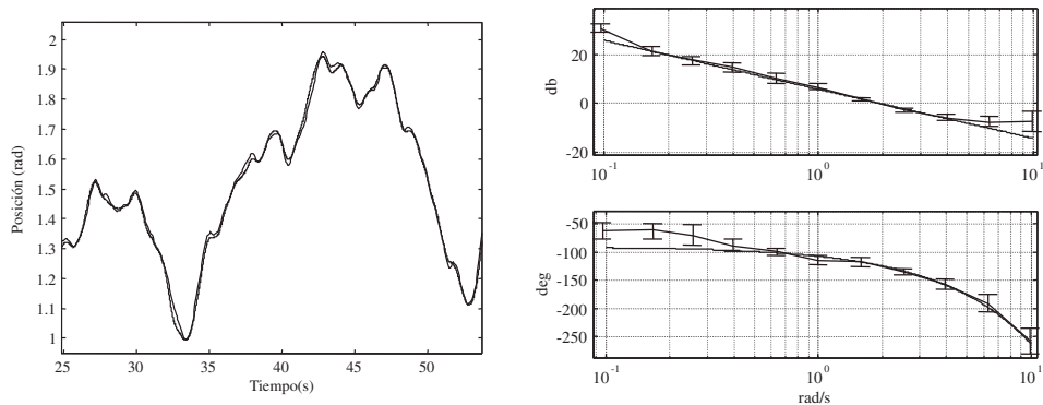
Figura 11.18. Comparación temporal y frecuencial entre la respuesta experimental (claro) y la respuesta del modelo de cross-over (oscuro) para un experimento de movimiento continuo utilizando un dispositivo de entrada de un grado de libertad.
