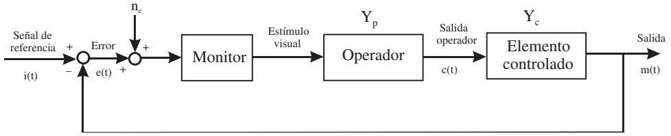
Figura 11.17. Sistema de teleoperación con visualizador compensatorio.
