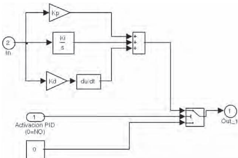
Figura 7.31. Bloque R(s) . Regulador PID.
