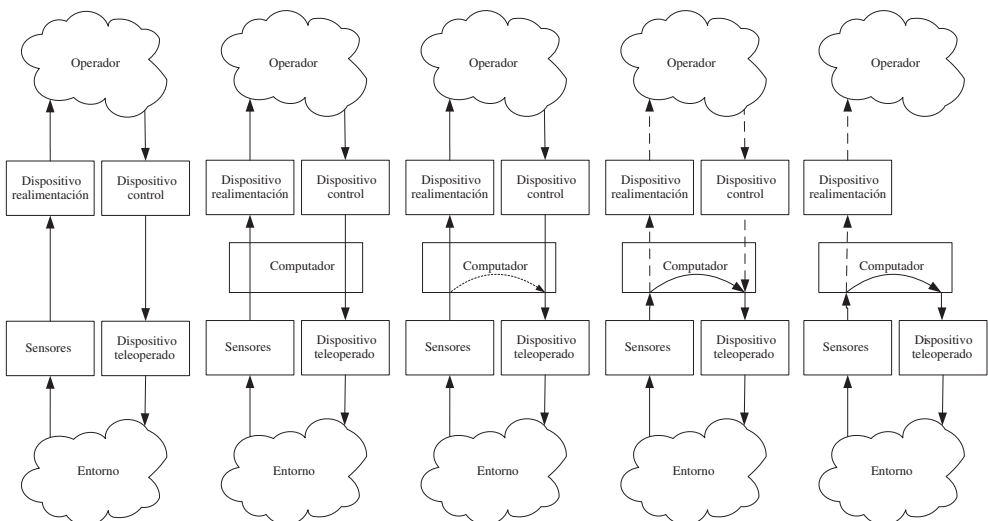
Figura 11.4. Niveles de modo de control remoto. Adaptado de [SHERIDAN-92].
