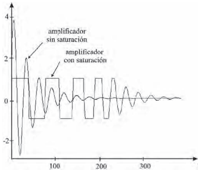
Figura 7.23. Comparación entre el par proporcionado por un amplificador con y sin saturación.
