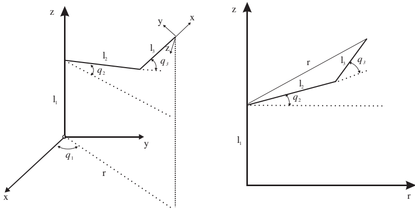
Figura 4.3. Robot de 3 grados de libertad.
