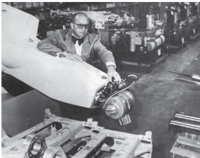
Figura 1.6. Joseph Engelberger con uno de los primeros Unimate.
