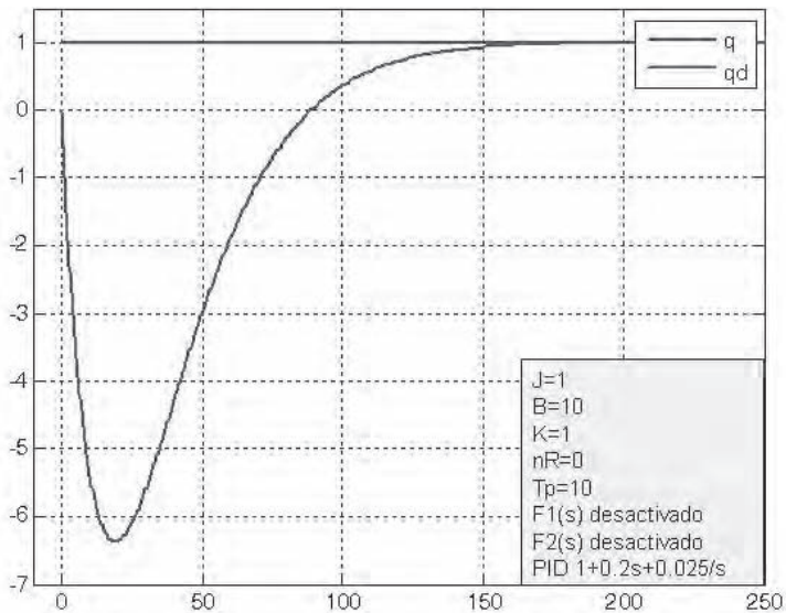
Figura 7.46. Trayectoria deseada q_d y real q , ante entrada escalón y perturbación T_p de 10 unidades con control PID.
