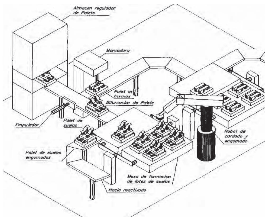
Figura 9.1. Ejemplo de lay-out de una célula robotizada de fabricación de calzado.
