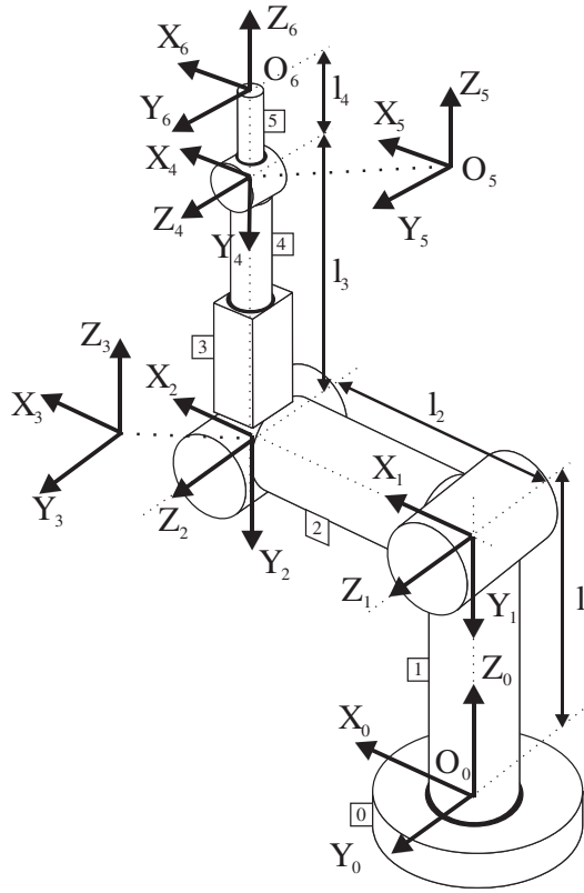
Figura 4.13. Cinemática del robot IRB2400, cuya inversa se puede desacoplar.
