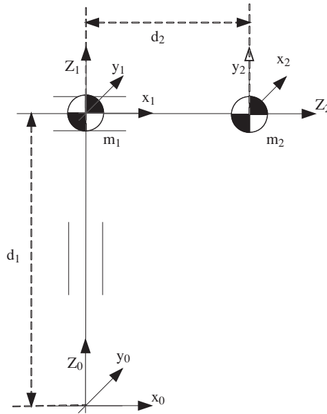
Figura 5.13. Robot cartesiano del Ejercicio 5.1.
