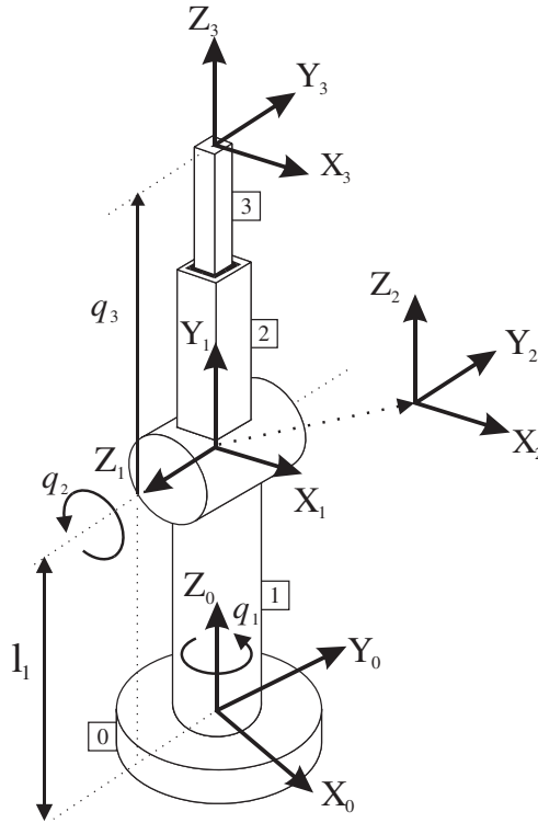
Figura 4.12. Asignación de sistemas de referencia del robot polar de la Figura 4.11.
