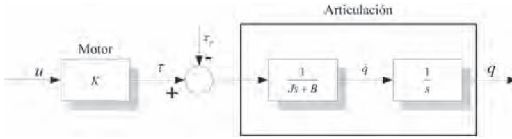
Figura 7.5. Diagrama de bloques de una articulación.
