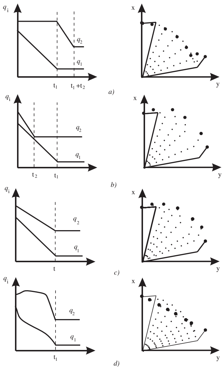
Figura 6.3. Diferentes trayectorias articulares posibles para un robot articular de 2 GDL. a) movimiento eje a eje, b) movimiento simultáneo de ejes, c) trayectoria coordinada, d) trayectoria continua rectilínea.
