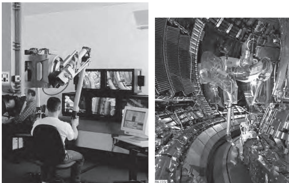
Figura 11.42. Imagen del sistema de teleoperación MASCOT instalado en el Joint European Torus-JET para su mantenimiento. (Cortesía de EFDA-JET).
