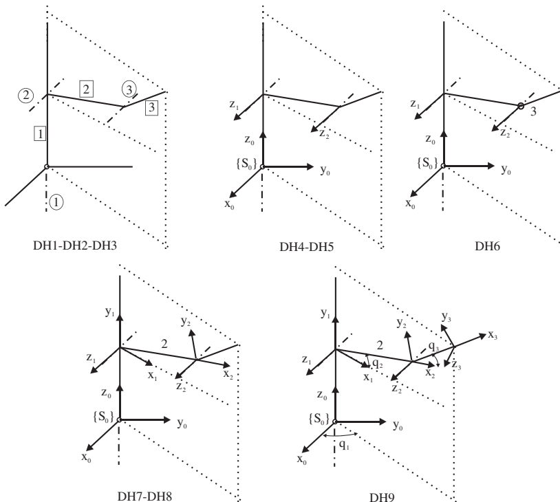
Figura 4.21. Secuencia del algoritmo de D-H para el robot del ejercicio 4.2.
