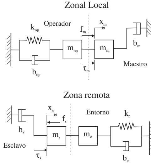
Figura 11.32. Modelo general de un sistema de teleoperación con control bilateral.
