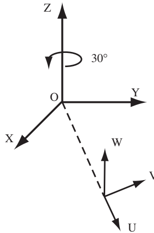
Figura 3.24. Figura Ejercicio 3.6.
