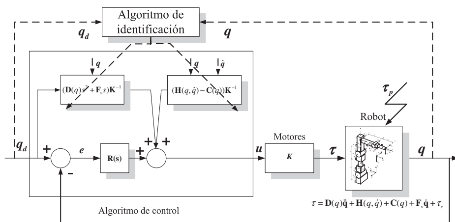
Figura 7.18. Esquema de control por par calculado adaptativo.
