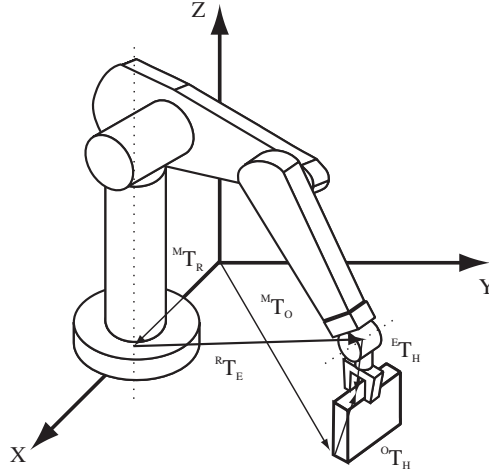
Figura 3.20. Ejemplo de aplicación de diversas transformaciones para localizar un objeto.
