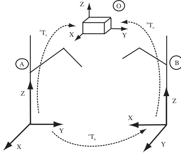
Figura 3.28. Matrices de transformaciones del Ejercicio 3.9.
