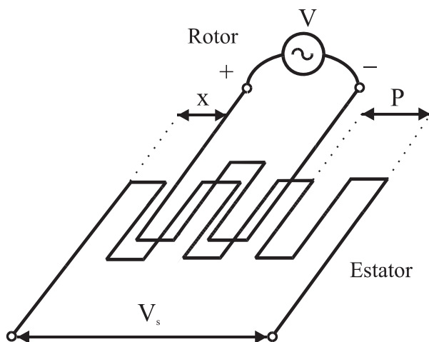
Figura 2.26. Esquema de funcionamiento de un Inductosyn.
