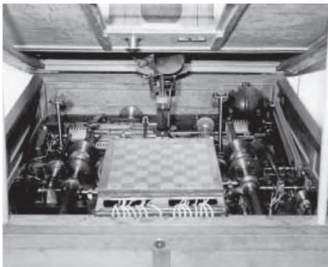
Figura 1.4. Máquina ajedrecista de Leonardo Torres Quevedo. (Cortesía del Museo Torres Quevedo).
