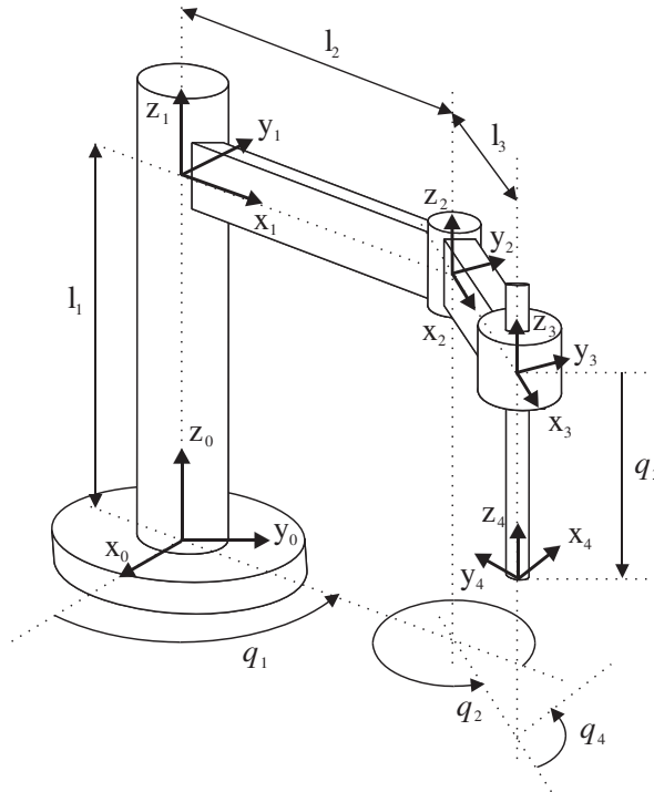
Figura 4.8. Asignación de los sistemas de referencia a un robot SCARA.
