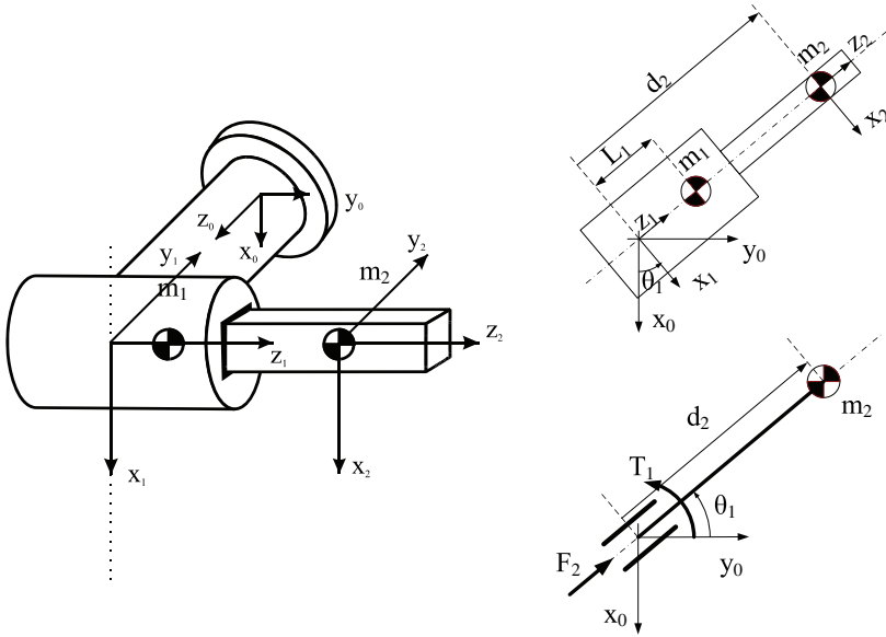
Figura 5.16. Robot Polar de 2 grados de libertad en disposición tumbada del Ejercicio 5.3.
