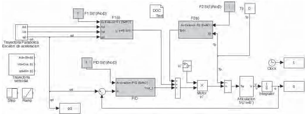
Figura 7.28. Esquema general de control monoarticular. Ejercicio 7.1.
