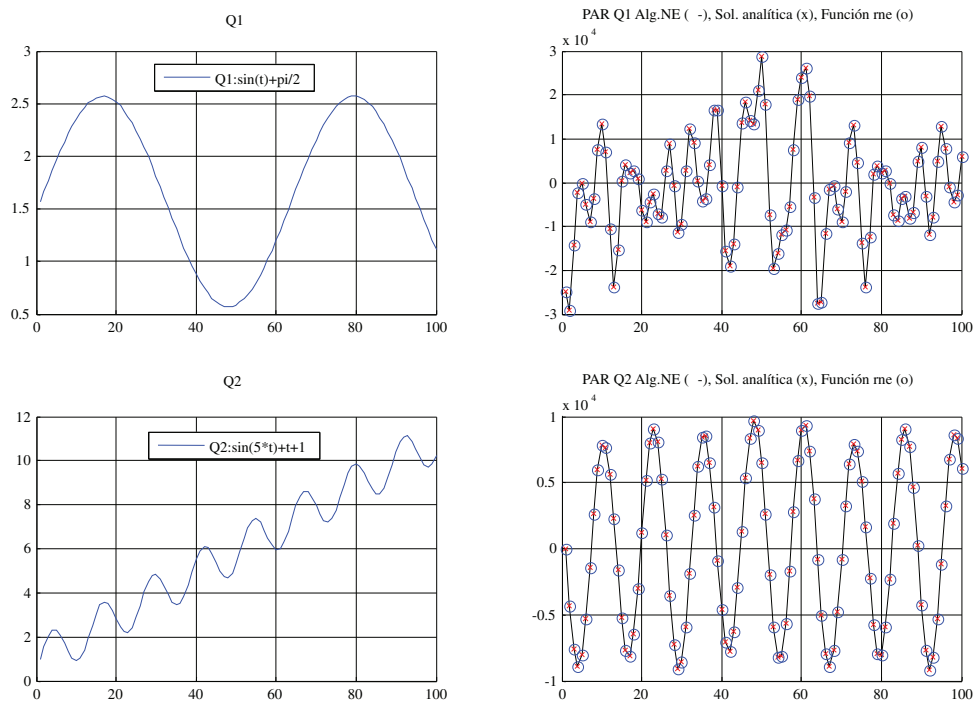
Figura 5.26. Trayectoria y Pares con los 2 gdl en movimiento.
