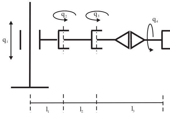
Figura 4.23. Figura del Ejercicio 4.3.
