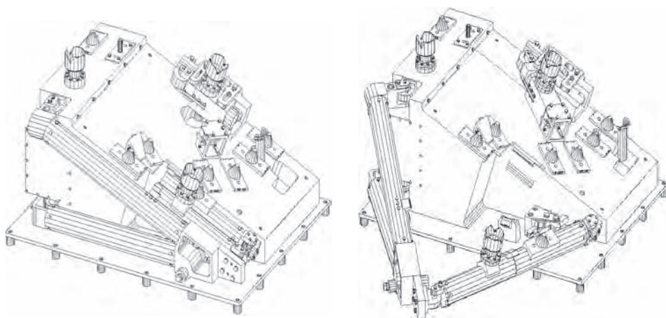
Figura 11.54. Configuración plegada (izquierda) y desplegada (derecha) de la estructura de despliegue sobre el TSE. (Cortesía de JAXA).
