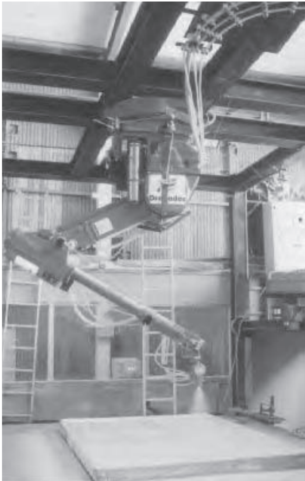
Figura 9.6. Robot IRB 3200 proyectando cemento en disposición suspendida. (Cortesía de DISAM-Universidad Politécnica de Madrid).
