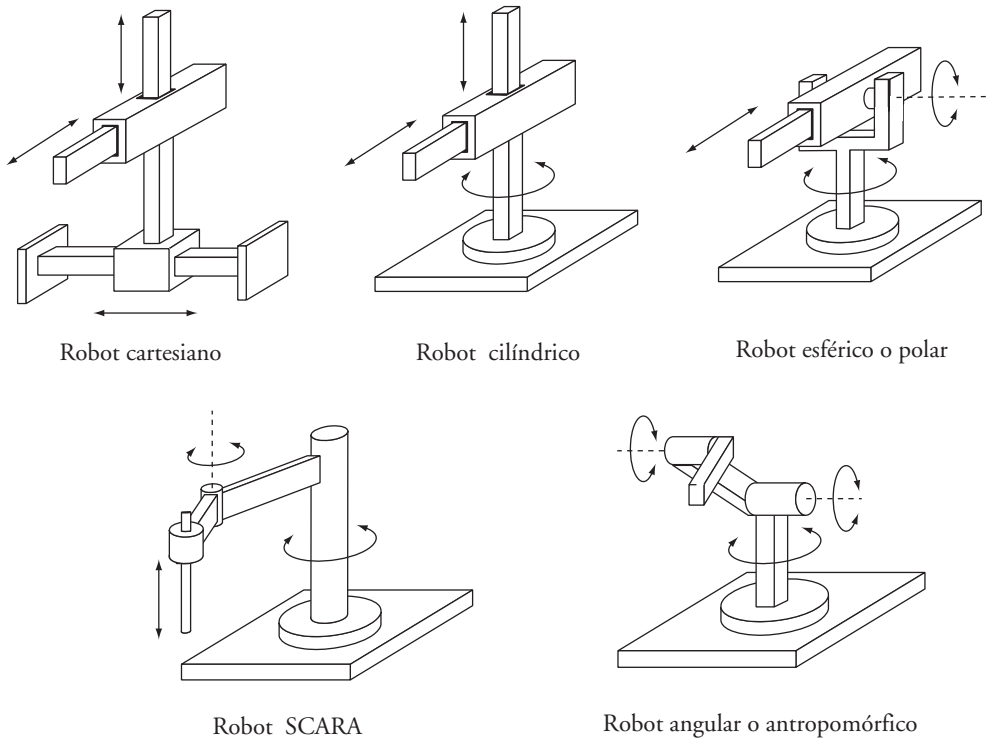
Figura 2.4. Configuraciones más frecuentes en robots industriales.
