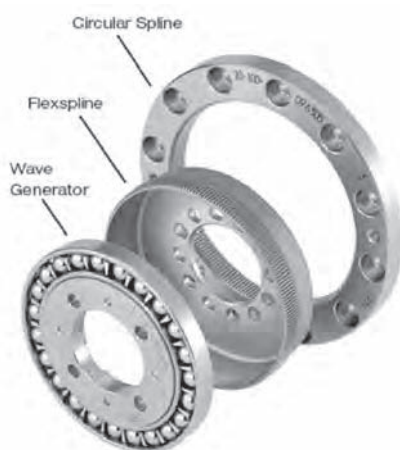
Figura 2.9. Despiece Reductor Armónico. (Cortesía Harmonic Drive).
