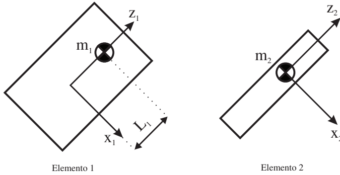
Figura 5.4. Elementos del robot polar del Ejemplo 5.1.
