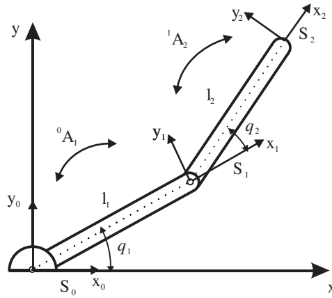
Figura 4.27. Robot Ejercicio 4.5.
