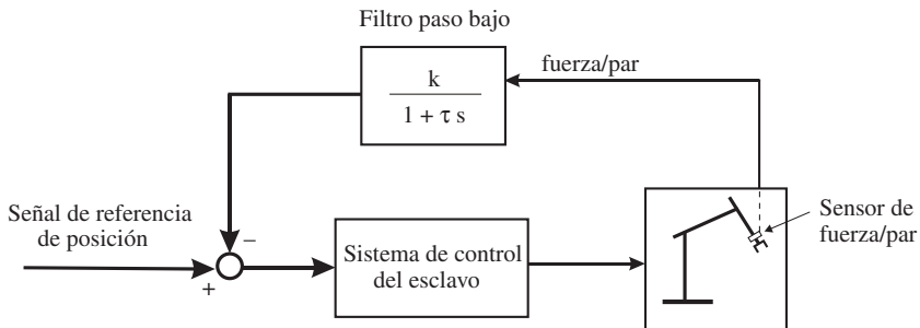
Figura 11.25. Esquema de implementación de la acomodación activa remota.
