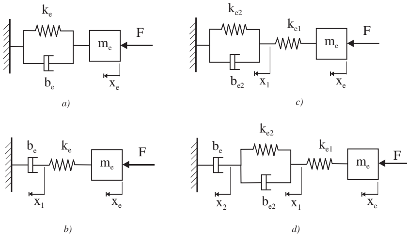
Figura 11.33. Modelos de entorno alternativos a) Kelvin, b) Maxwell, c) lineal estándar y sólido y d) Maxwell-Kelvin.
