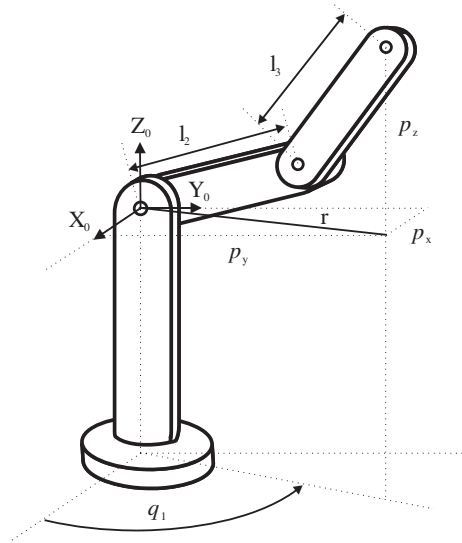
Figura 4.9. Robot articular.
